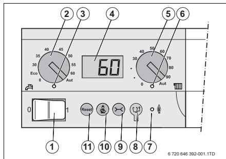
Bild 4 Bedienfeld – Bedienelemente
