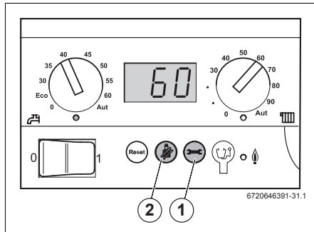
Bild 6 Bedieneinheit
