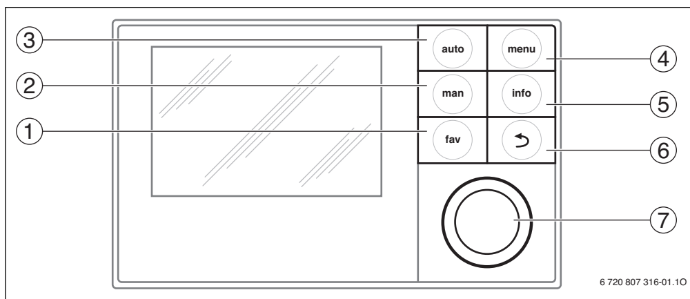
Bild 1 Bedienelemente
