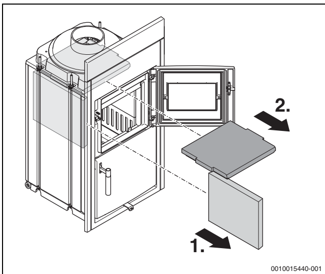
Bild 21 Feuerraumauskleidung ausbauen
