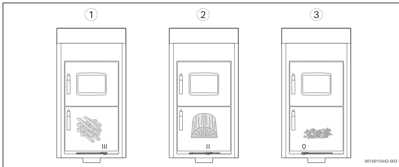
Bild 24 Verbrennungsluftschieber-Stellungen
