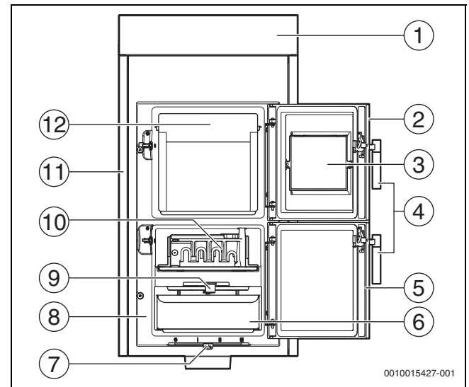
Bild 3 Produktübersicht
