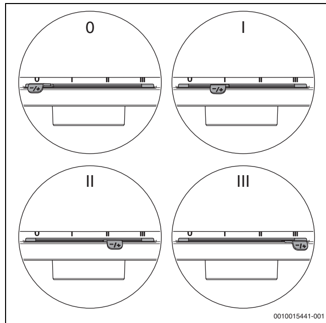
Bild 23 Verbrennungsluftschieber regulieren
