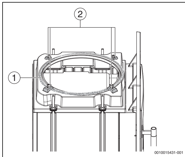
Bild 7 Kuppel montieren
