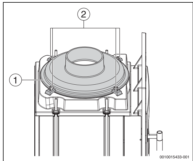
Bild 9 Kuppel senkrecht
