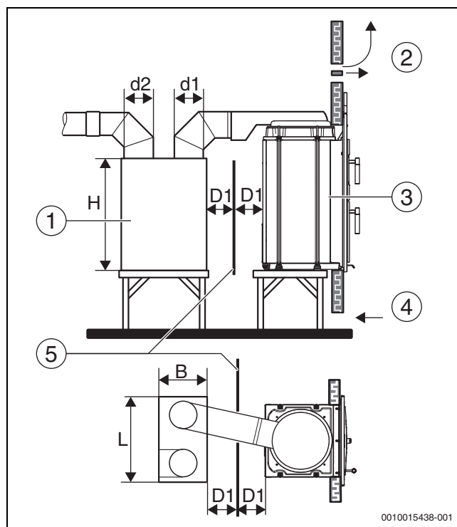
Bild 15 Heizeinsatz mit waagerechter Kuppel (schematische Darstellung)
