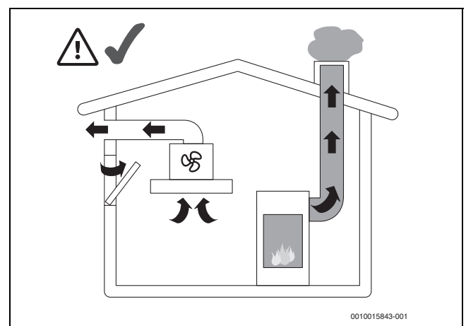
Bild 2 Richtiger Weg der Frischluftzufuhr
