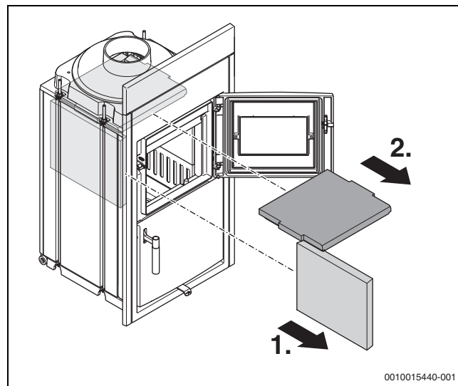
Bild 14 Feuerraumauskleidung ausbauen
