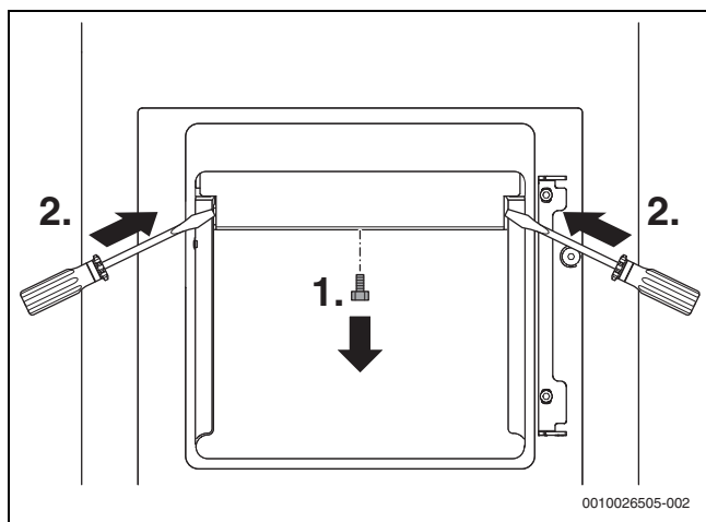
Bild 11 Sicherungsschraube entfernen und Isolierstein nach hinten drücken
