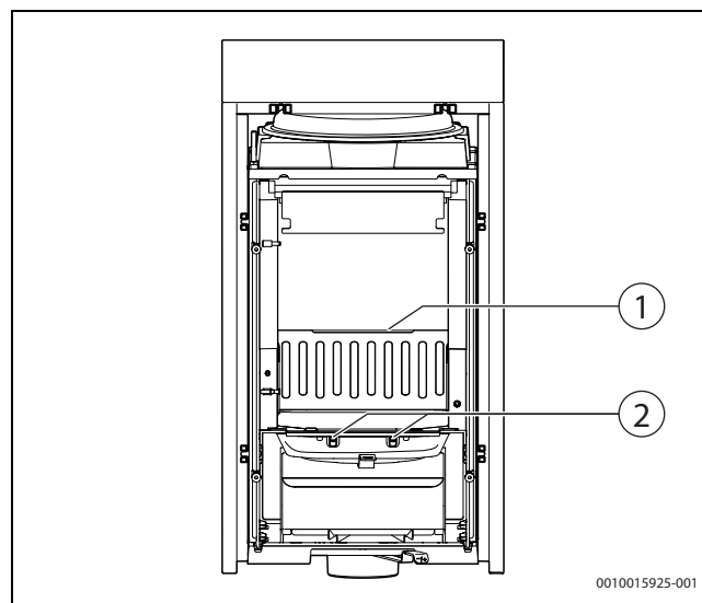
Bild 10 Luftöffnungen
