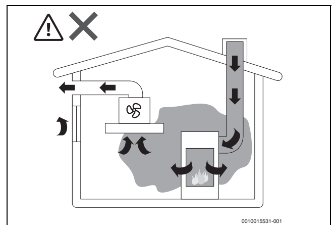
Bild 1 Falscher Weg der Frischluftzufuhr
