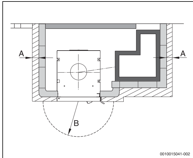
Bild 5 Äußere Mindestabstände
