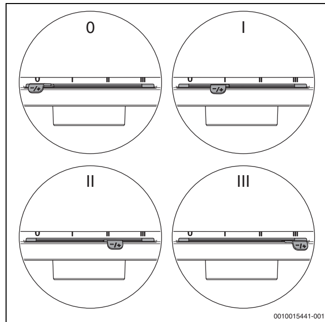
Bild 8 Verbrennungsluftschieber regulieren
