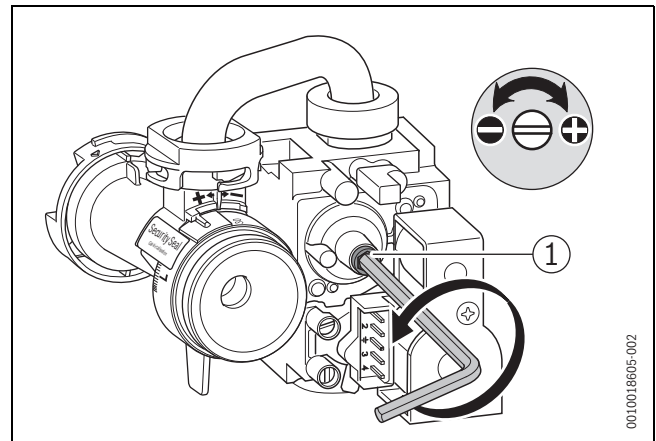
Bild 64 Plombe entfernen
