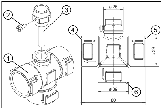
Blind 1: Kreuzstück
