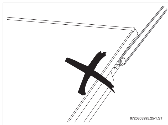
Bild 15 Kollektoranschlüsse nicht als Transporthilfe nutzen
