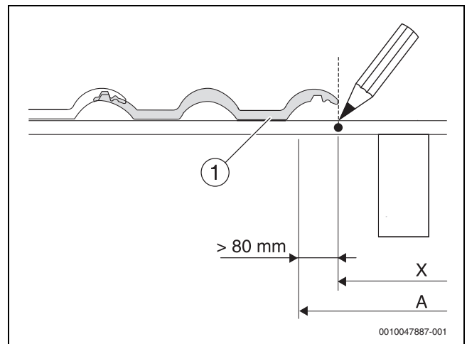
Bild 19 Maß X
