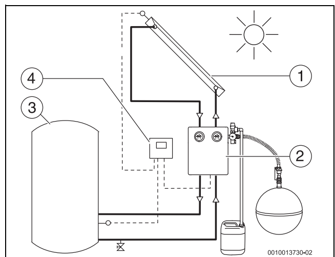
Bild 9 Beispielhafte Darstellung einer Solaranlage
