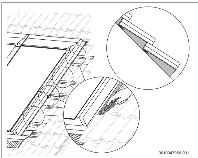
Bild 74 Dreieckdichtband einschneiden
