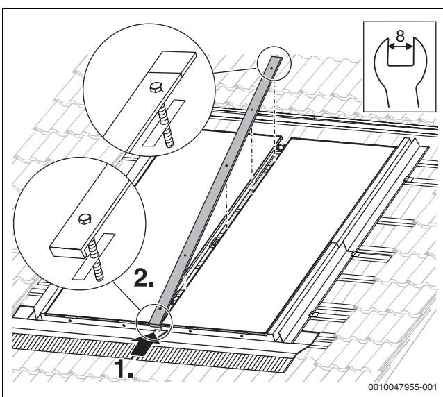
Bild 64 Abdeckleiste montieren
