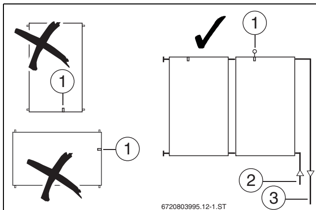
Bild 11 Anordnung senkrechter und waagrecht Kollektoren
