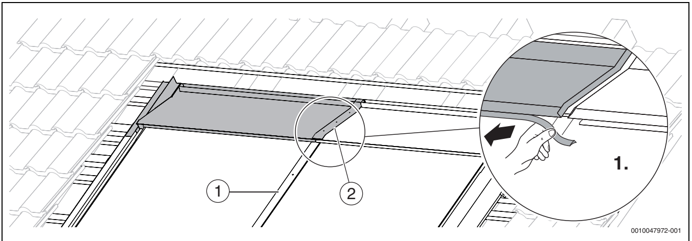
Bild 81 Dichtlippe abziehen
