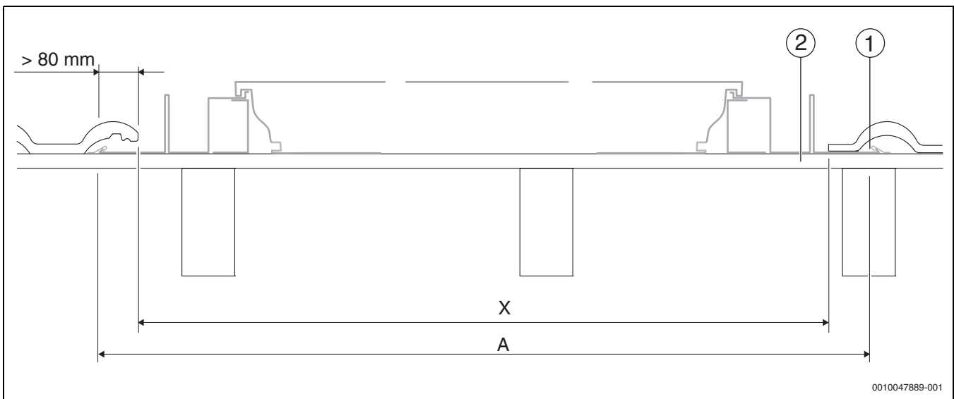
Bild 21 Kollektorfeldbreite
