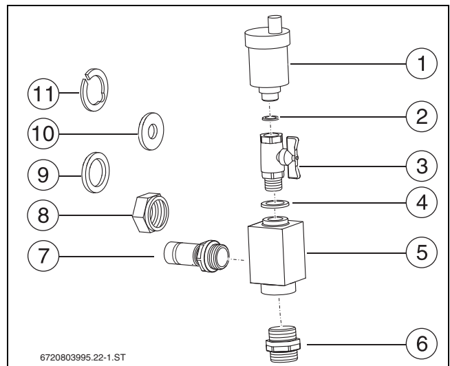
Bild 55 Lieferumfang Entlüfter-Set
