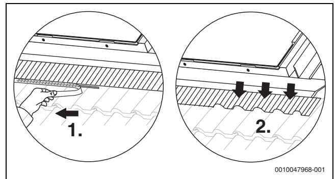
Bild 76 Bleischürzen auf Eindeckung kleben
