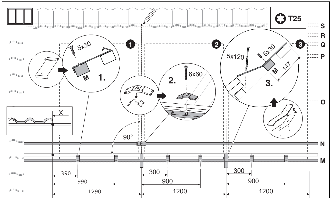
Bild 27 Kolleortyp senkrecht (3 Kollektoren), Maße in mm
