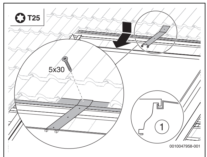
Bild 67 Waagerechte Ausführung
