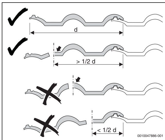
Bild 18 Im Wellental schneiden und mindestens halbe Dachziegel stehen lassen
