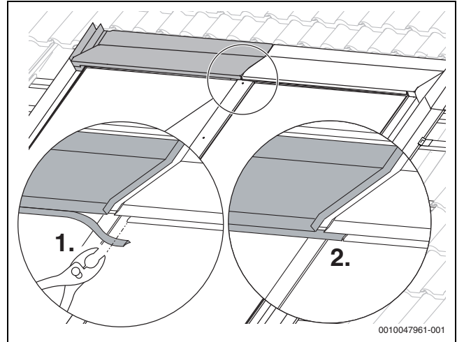
Bild 70 Dichtlippe anpassen
