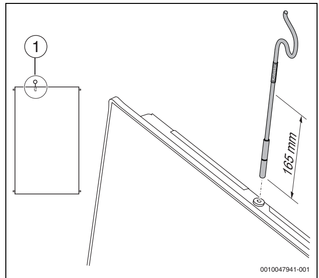
Bild 51 Kollektorfühler montieren
