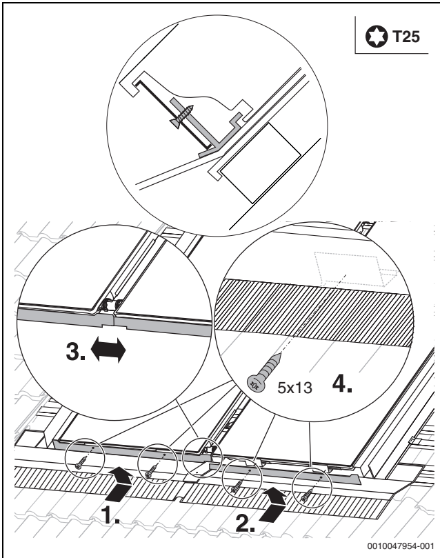
Bild 63 Blenden festschrauben
