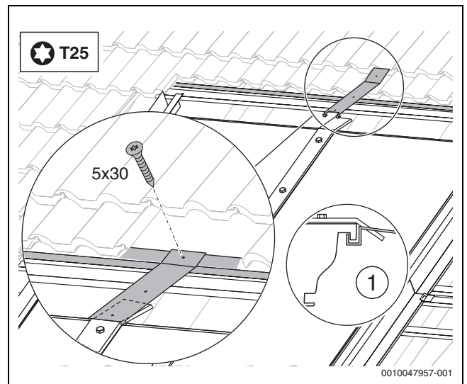
Bild 66 Senkrechte Ausführung
