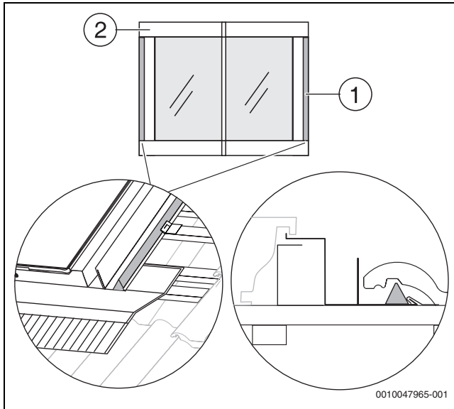
Bild 73 Dreieckdichtband einlegen
