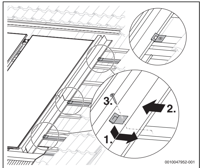
Bild 61 Hafter montieren
