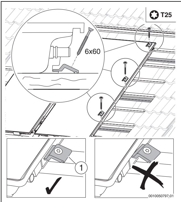
Bild 49 Niederhalter festschrauben
