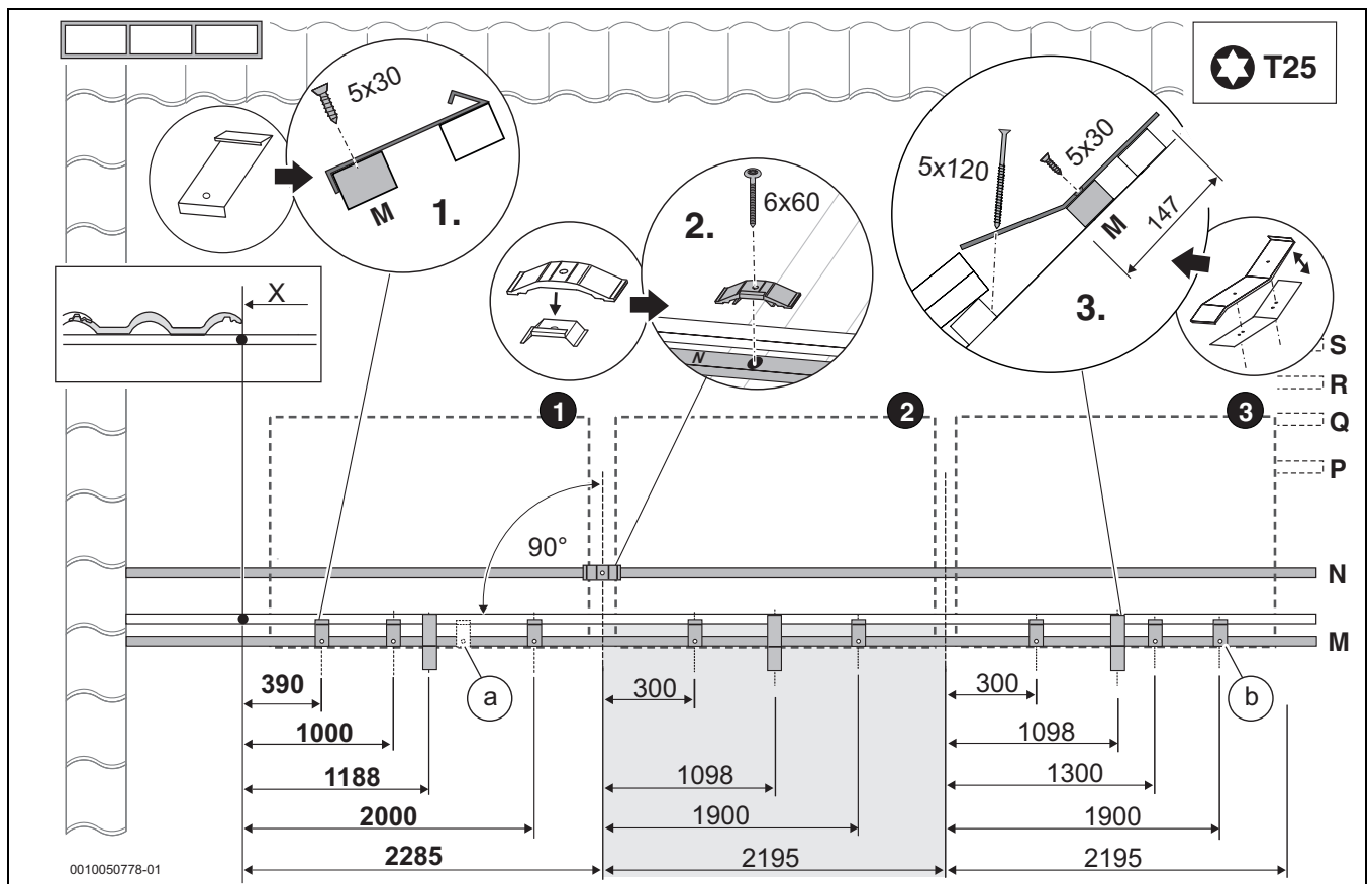
Bild 28 Kolleortyp waagrecht (3 Kollektoren), Graubereich: bei mehr als 2 Kollektoren (diese Maße wiederholen sich), Maße in mm
