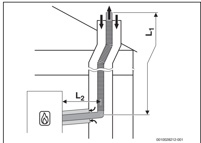
Bild 14 Flexible Abgasführung nach C 93x im Schacht und konzentrische Luft-Abgas-Führung im Aufstellraum
