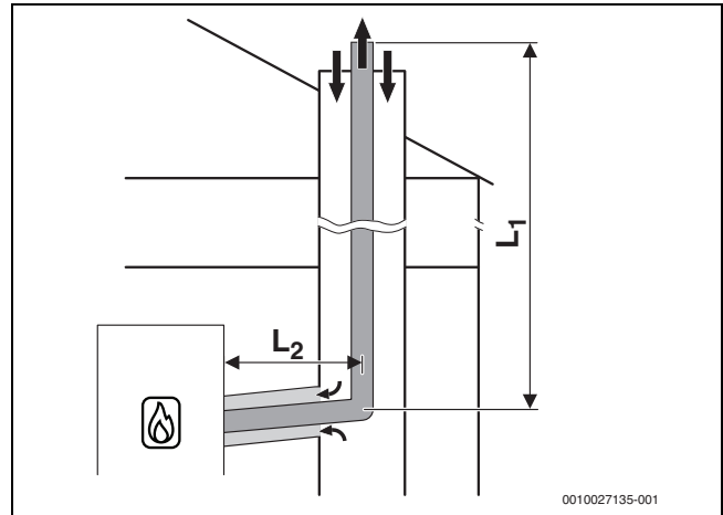
Bild 13 Starre Abgasführung nach C 93x im Schacht und konzentrische Luft-Abgas-Führung im Aufstellraum
