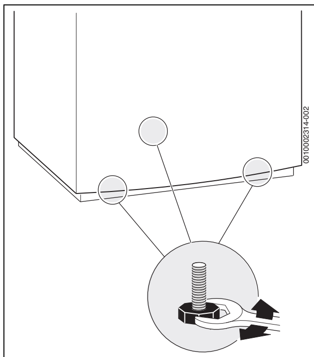
Bild 49 Speicher ausrichten
