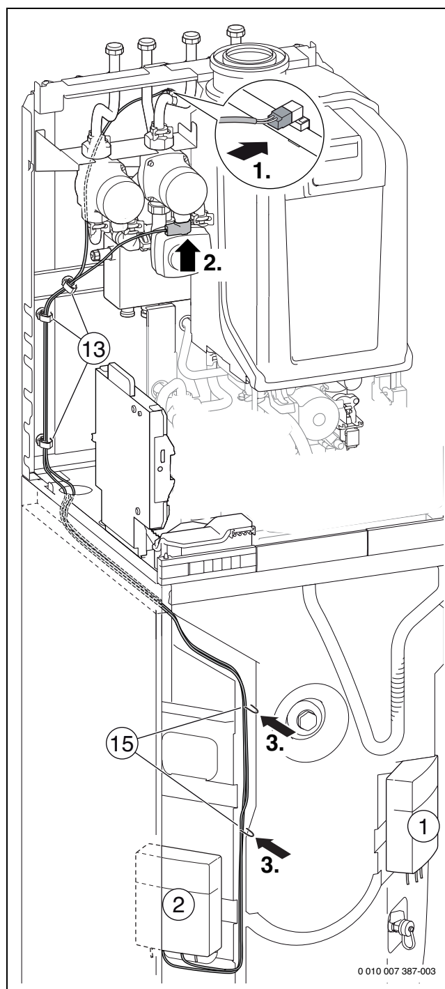
Bild 132 Anschluss Heizungspumpe gemischter Heizkreis und Temperaturfühler
