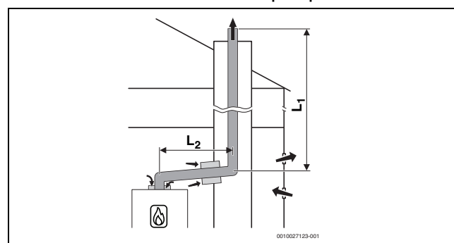
Bild 31 Starre Abgasführung im Schacht nach B 23p /B 53p mit raumluftabhängiger Luftzufuhr am Gerät und konzentrischem Verbindungsstück zwischen Aufstellraum und Schacht
