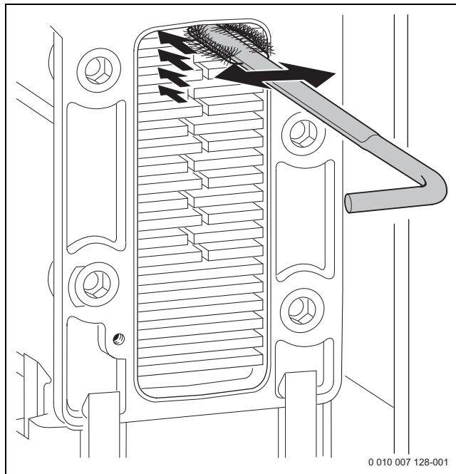
Bild 205 Wärmeblock mit Bürste reinigen
