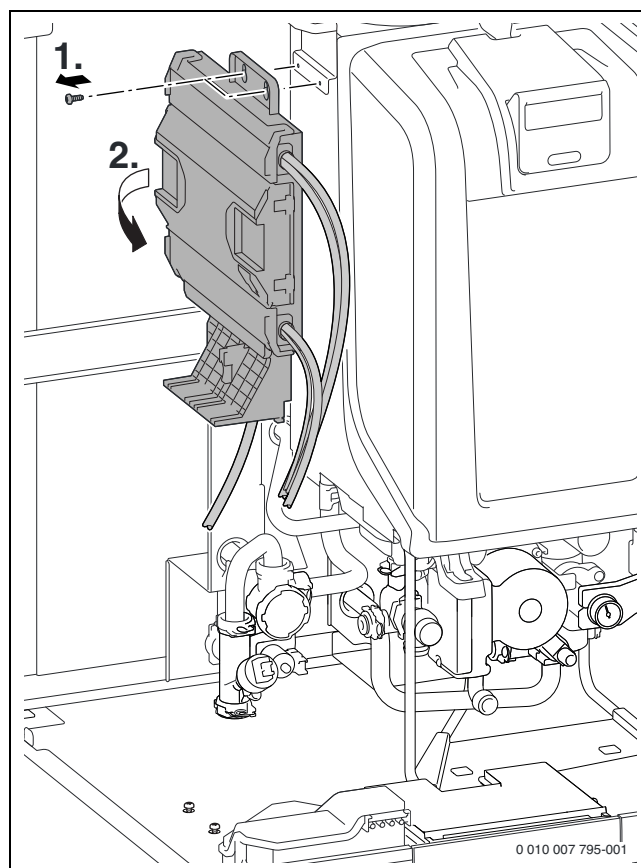
Bild 58 Steuergerät abnehmen
