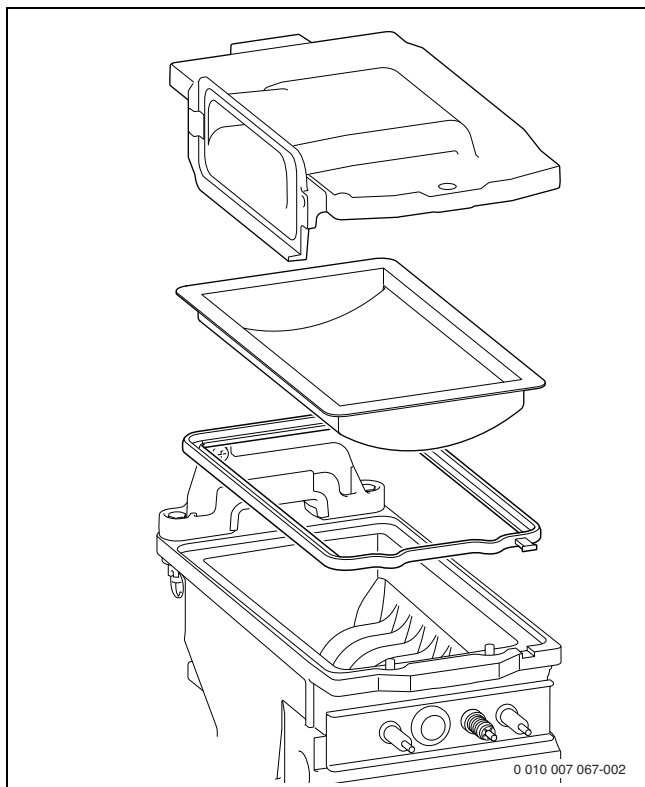
Bild 203 Brenner
