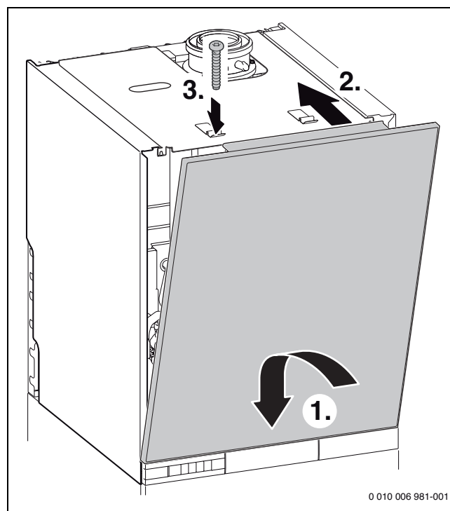
Bild 188 Vordere Verkleidung einhängen und mit Schraube aus Lieferumfang sichern
