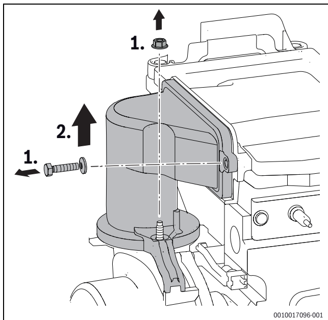
Bild 210 Mischeinrichtung ausbauen
