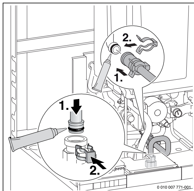
Bild 57 Rohrverbindung zwischen Speicherrücklauf und Wärmeblock erstellen
