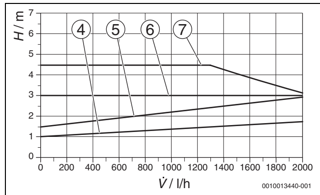
Bild 226 Pumpenkennlinien für Proportionaldruck und Konstantdruck
