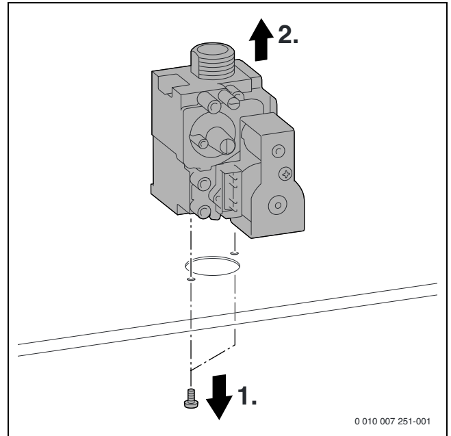
Bild 215 Gasarmatur ausbauen
