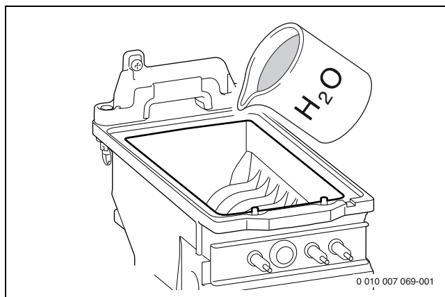
Bild 206 Spülen
