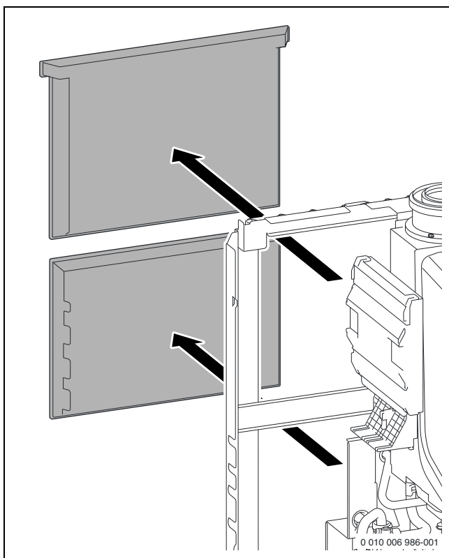
Bild 67 Wärmedämmungen an der Rückseite abnehmen
