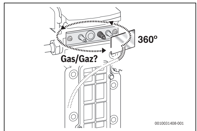
Bild 201 Dichtheit kontrollieren
