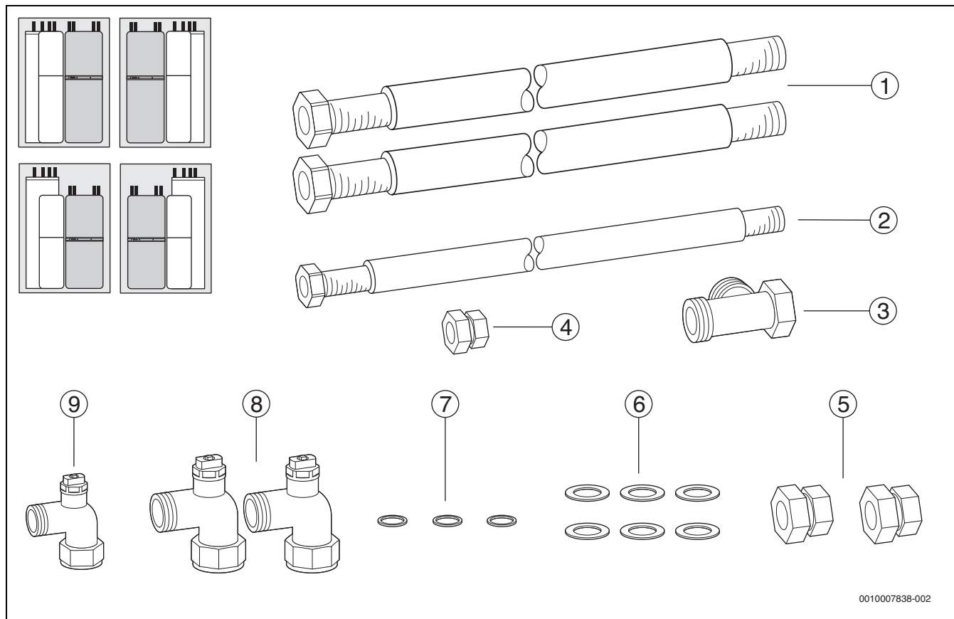
Bild 169 Lieferumfang
