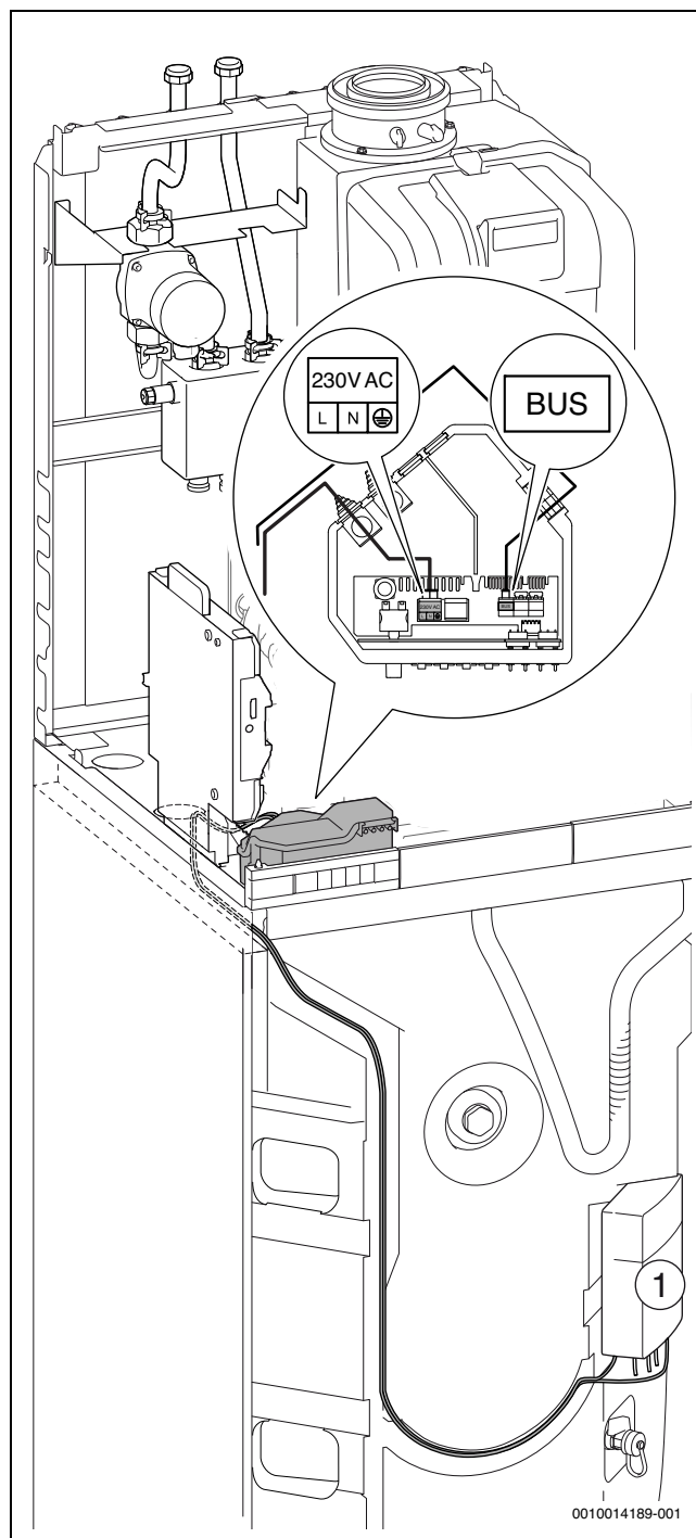
Bild 107 Anschluss Modul MM100
