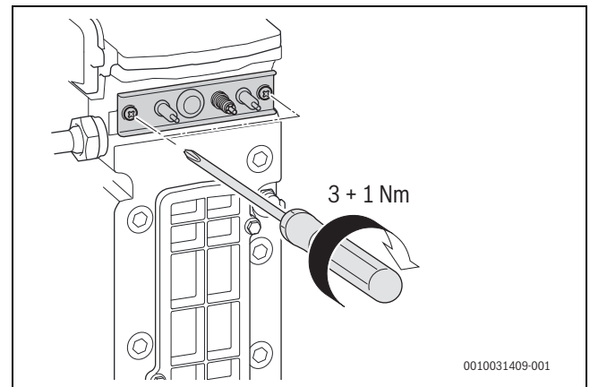
Bild 200 Elektroden-Set wieder einbauen
