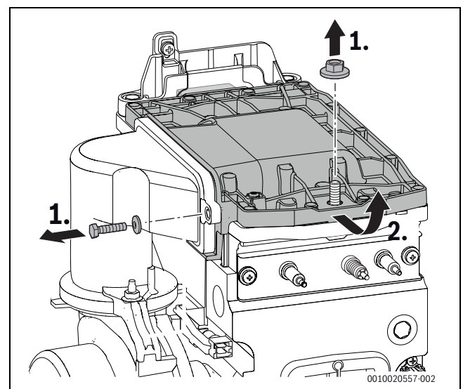
Bild 202 Brennerdeckel ausbauen
