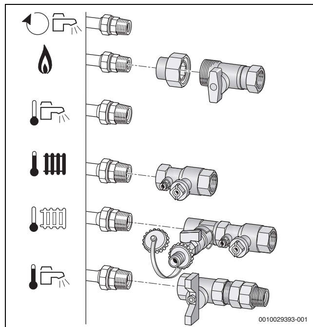
Bild 46 Montage des Armaturen-Sets am Beispiel Anschlüsse nach rechts AS-H1/Horizontales Anschluss-Set
