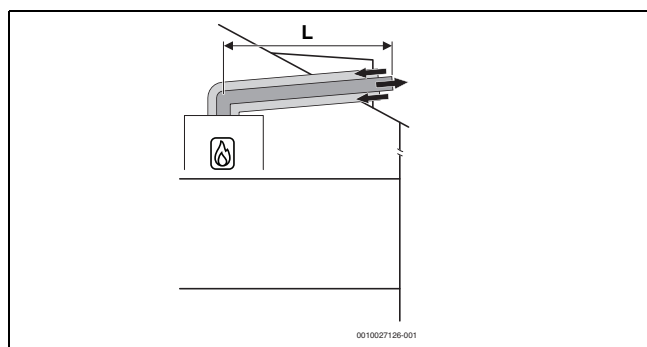
Bild 22 Horizontale konzentrische Luft-Abgas-Führung nach C 13x über das Dach
