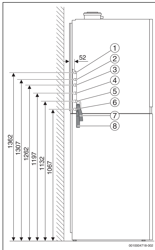
Bild 6 Anschlussmaße des Zubehörs AS-H1/Horizontales Anschluss-Set (Maße in mm)
