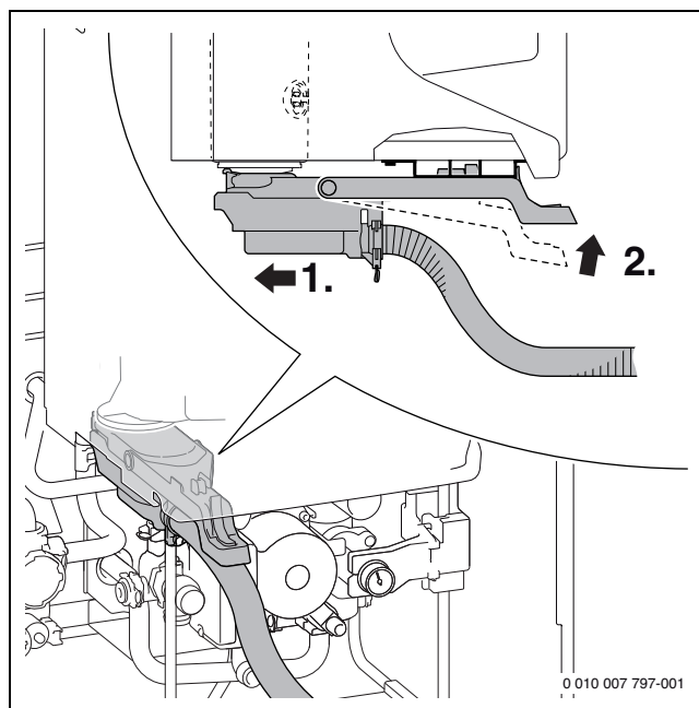
Bild 53 Schmutzfänger montieren
