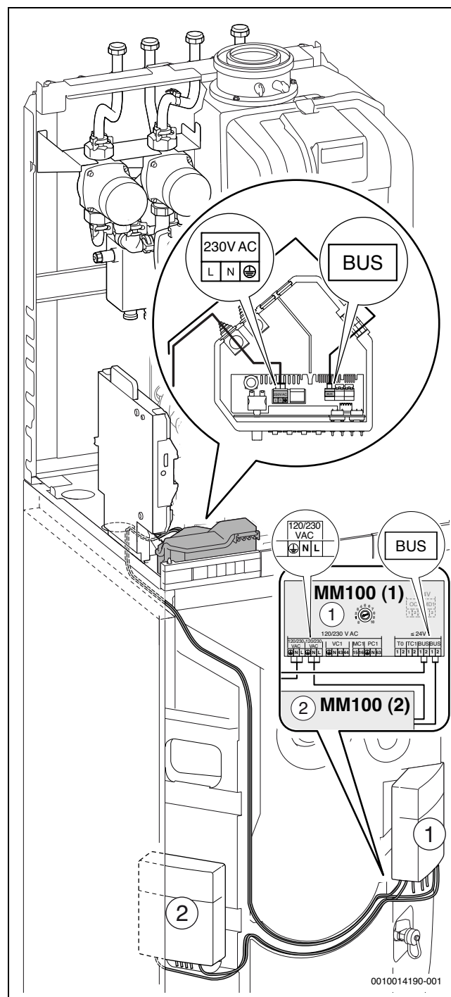
Bild 136 Anschluss MM100 (1) und MM100 (2)
