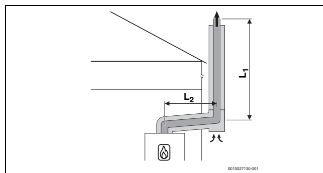
Bild 28 Konzentrische Luft-Abgas-Führung nach C 53x an der Außenwand
