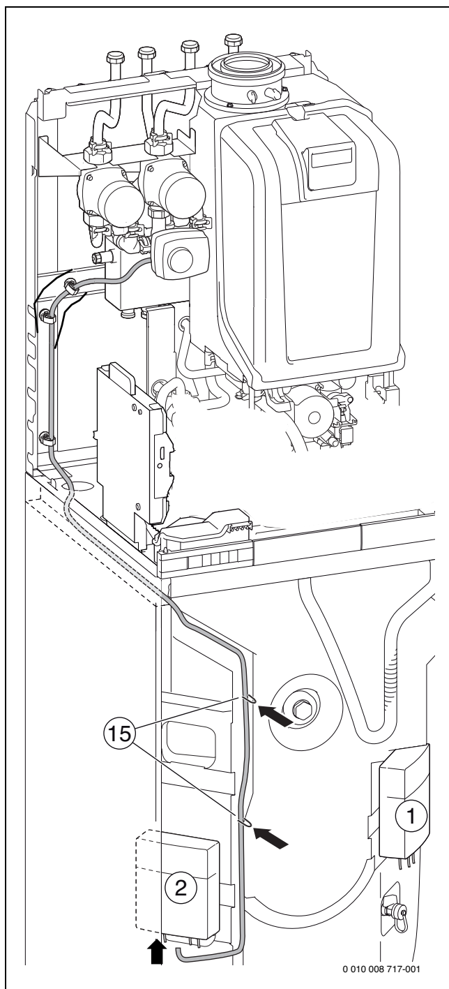
Bild 133 Anschluss Mischermotor
