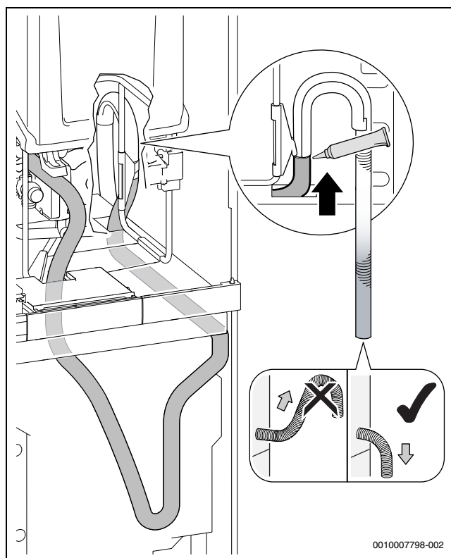
Bild 54 Siphonschlauch am Endstück einstecken
