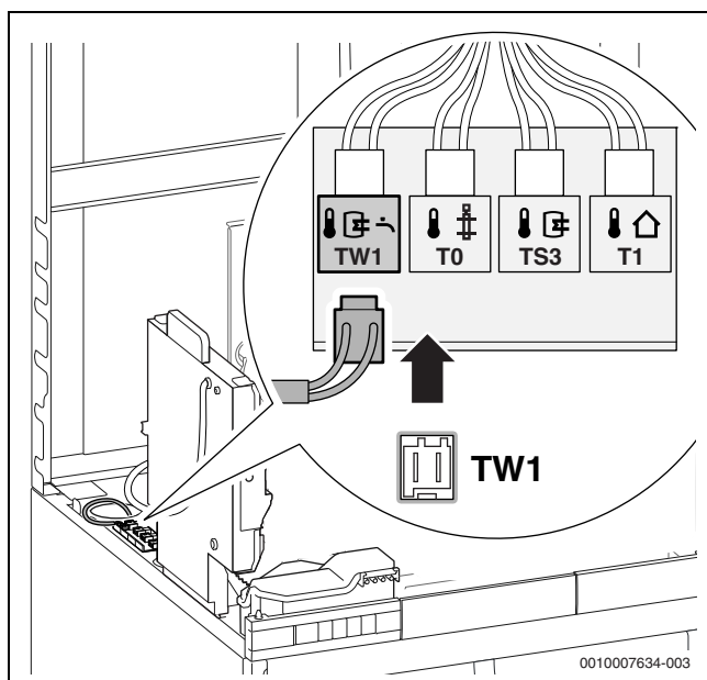
Bild 61 Speichertemperaturfühler anschließen
