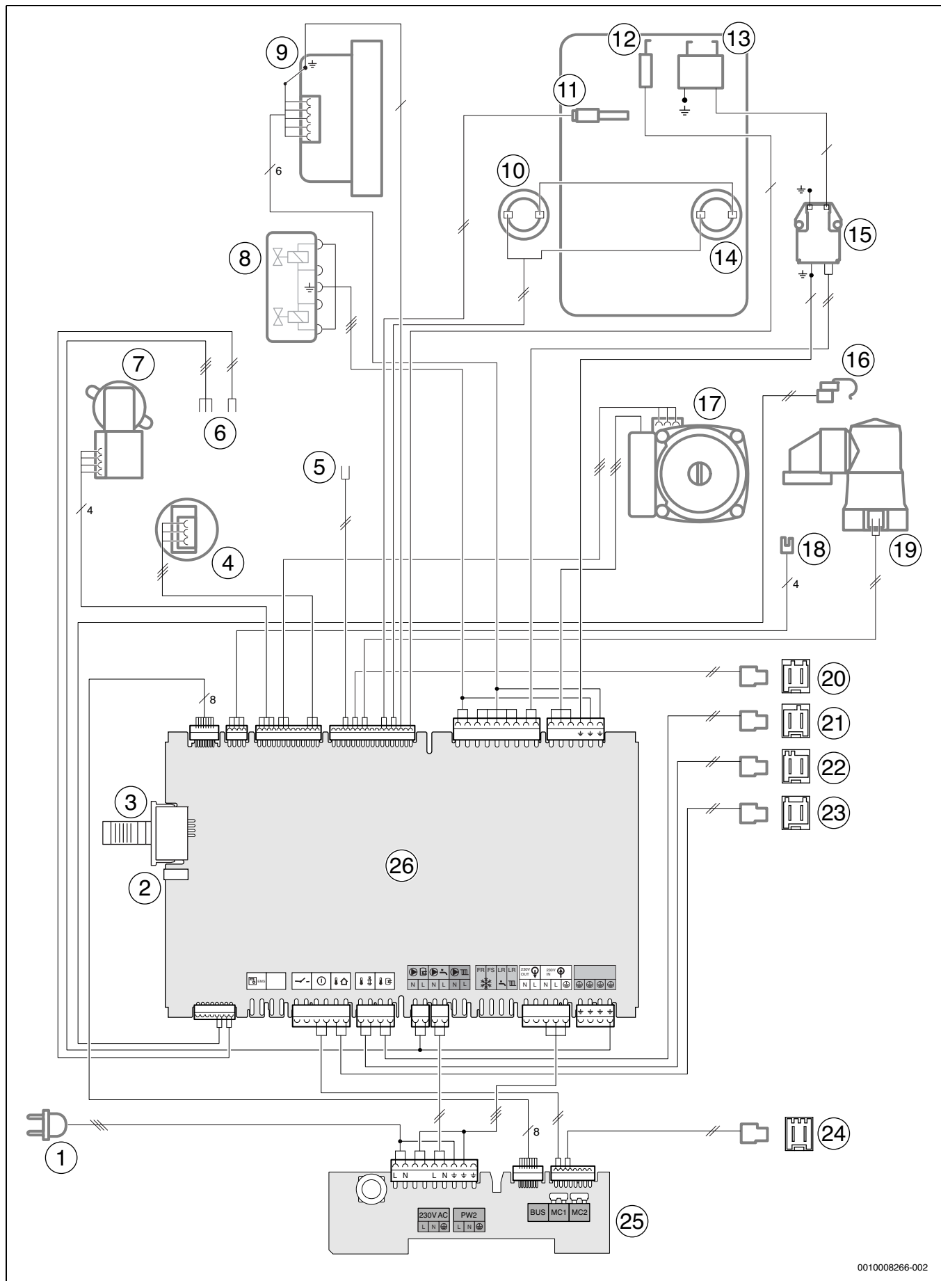
Bild 219 Elektrische Verdrahtung
