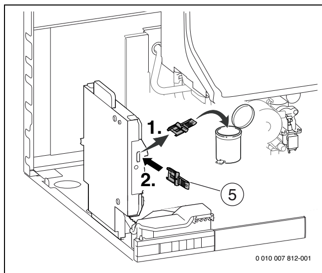
Bild 152 KIM tauschen
