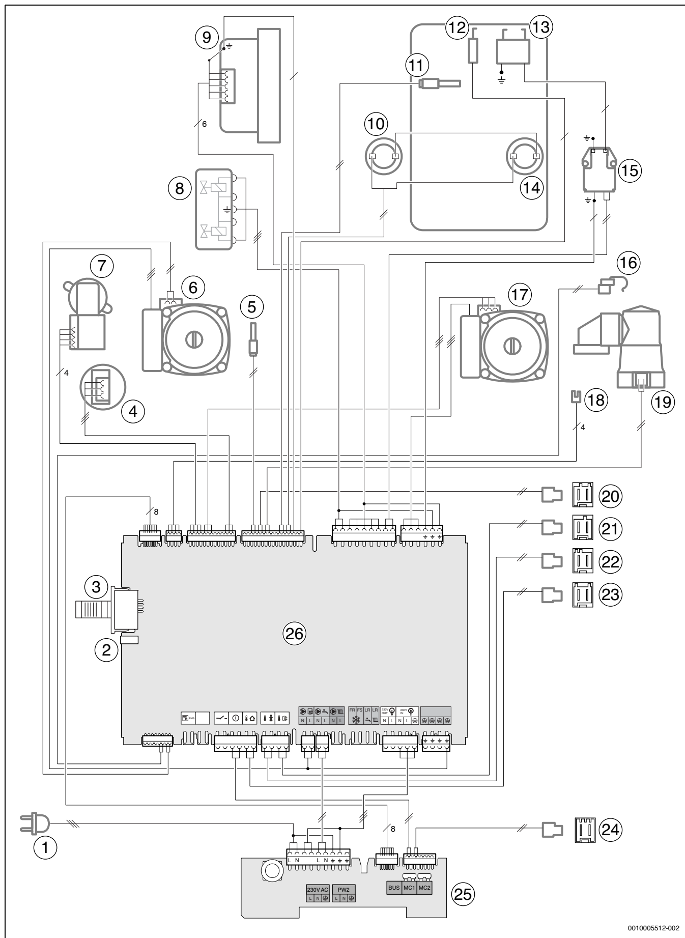
Bild 273 Elektrische Verdrahtung
