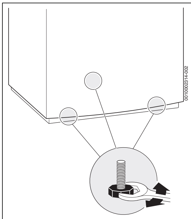
Bild 53 Speicher ausrichten
