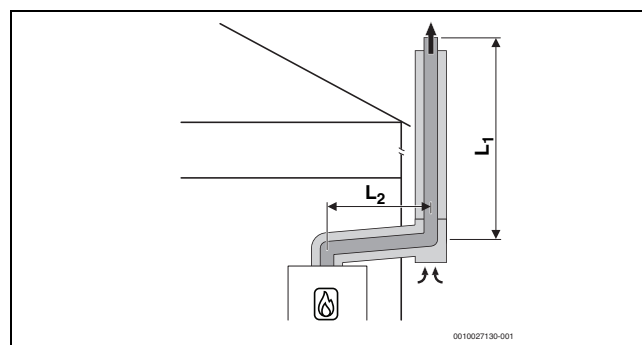
Bild 31 Konzentrische Luft-Abgas-Führung nach C 53x an der Außenwand
