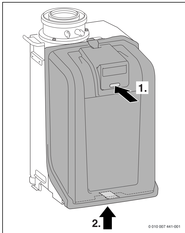
Bild 246 Brennerhaube abnehmen
