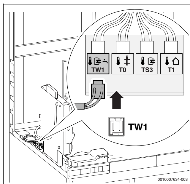
Bild 66 Speichertemperaturfühler anschließen
