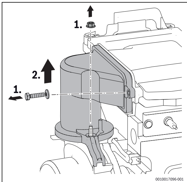
Bild 262 Mischeinrichtung ausbauen
