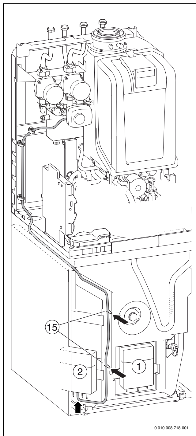
Bild 144 GB.192...iT100...-Geräte: Anschluss Mischermotor
