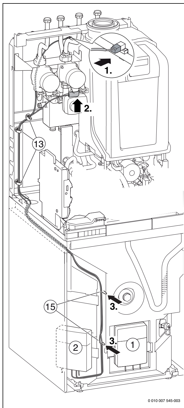
Bild 142 GB.192-..iT100-.-Geräte: Anschluss Heizungspumpe gemischter Heizkreis und Temperaturfühler
