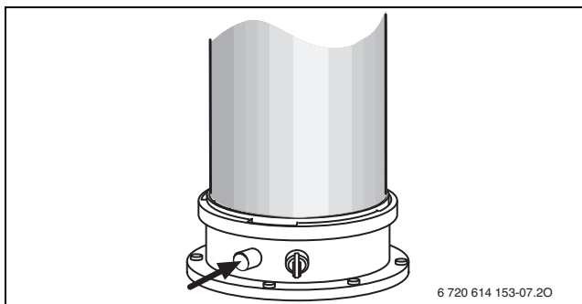
Bild 248 Abgasmessstutzen
