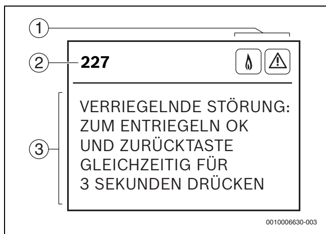
Bild 270 Störungsamenü
