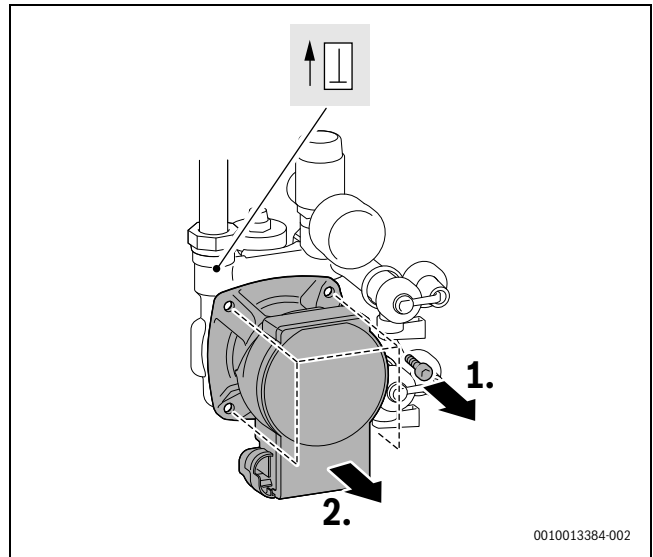
Bild 269 Solarpumpe ausbauen
