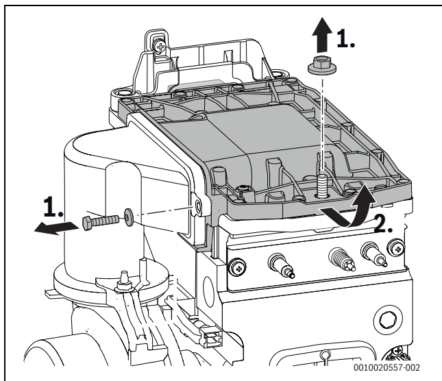
Bild 254 Brennerdeckel ausbauen
