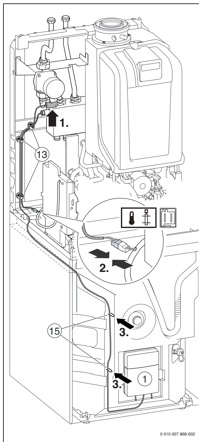
Bild 112 GB.192-..iT100-.-Geräte: Anschluss Heizungspumpe ungemischter Heizkreis und Hydraulische Weiche
