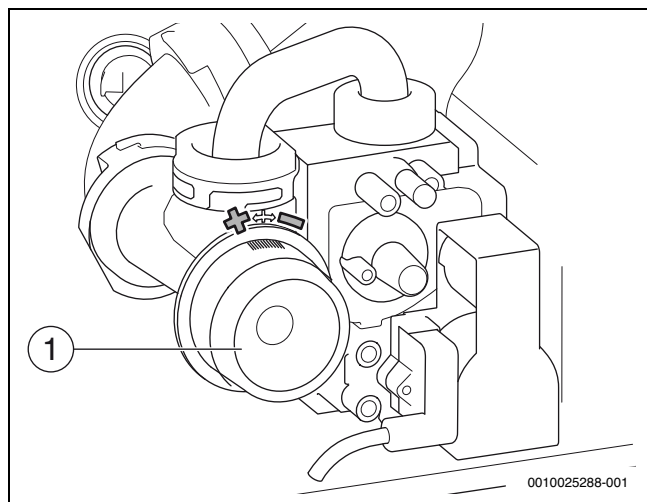
Bild 247 Gas-Luft-Verhältnis einstellen
