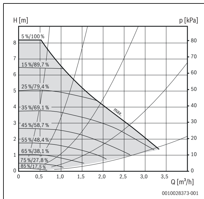
Bild 275 Pumpenkennfelder und Pumpenkennlinien der Solarpumpe Wilo Para ST 15/7-50/iPWM 2, Drehzahlbereich 20–100 %, Volumenstrombereich 0–16,5 l/min
