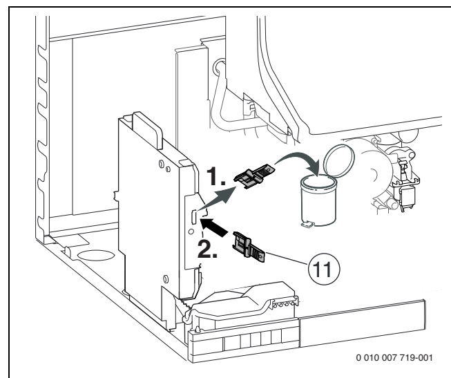
Bild 162 KIM tauschen
