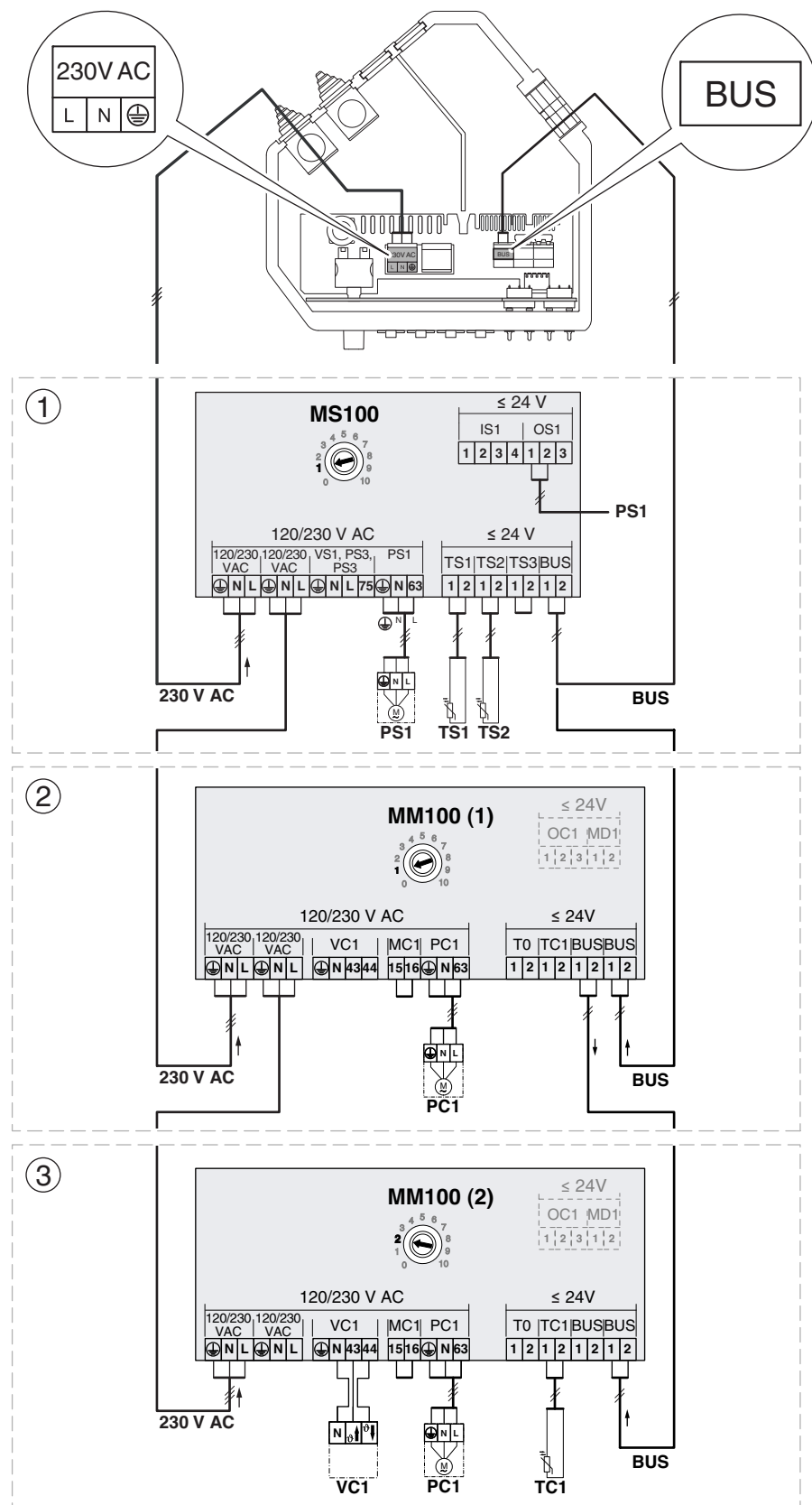
Bild 229 Anschluss der Module MS100 und MM100, wenn vorhanden
