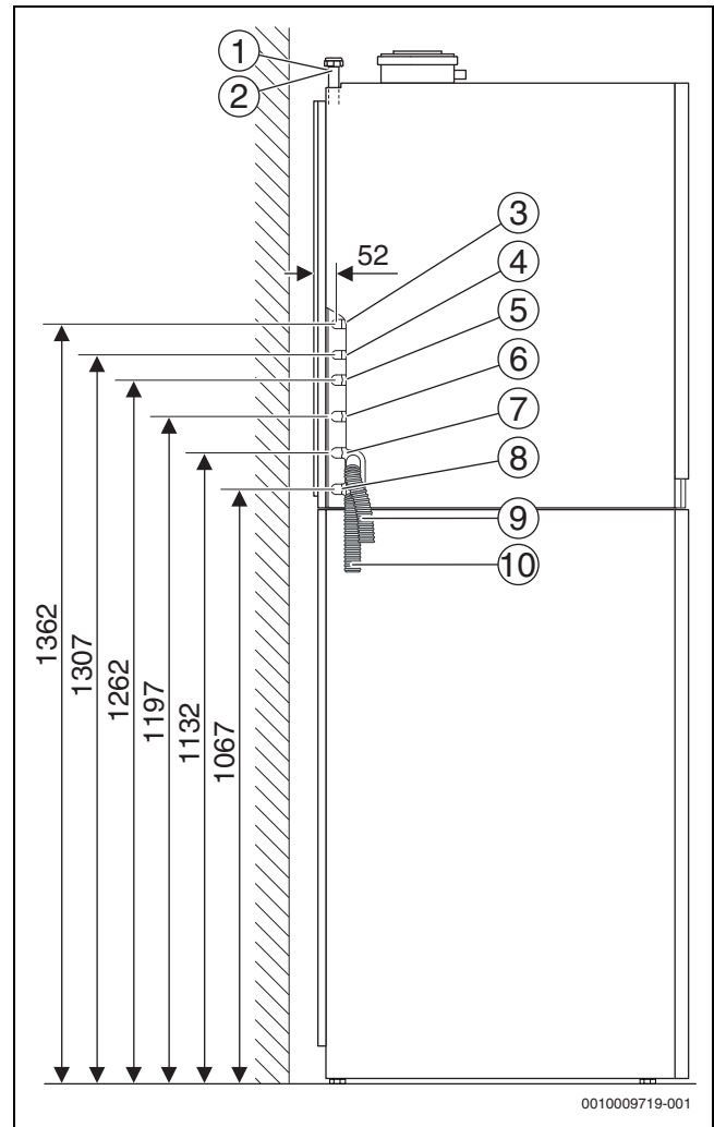
Bild 4 Anschlussmaße des Zubehörs AS-H1/Horizontales Anschluss-Set (Maße in mm)
