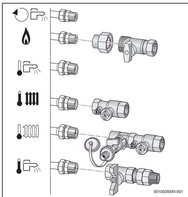
Bild 42 Montage des Armaturen-Sets am Beispiel Anschlüsse nach rechts AS-H1/Horizontales Anschluss-Set
