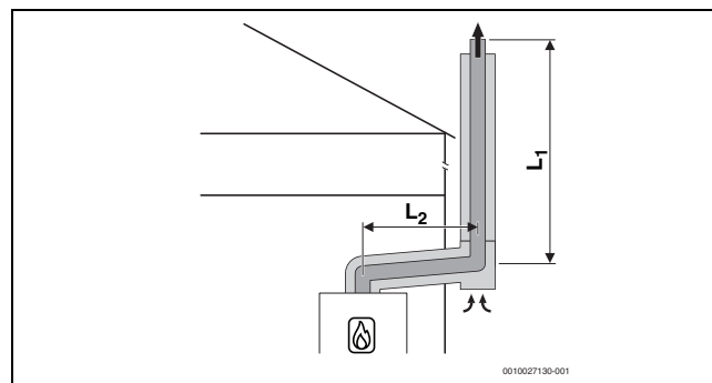
Bild 24 Konzentrische Luft-Abgas-Führung nach C 53x an der Außenwand
