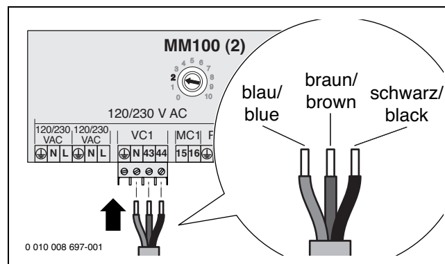
Bild 140 Anschluss Kabel Mischermotor am Modul MM100 [2]
