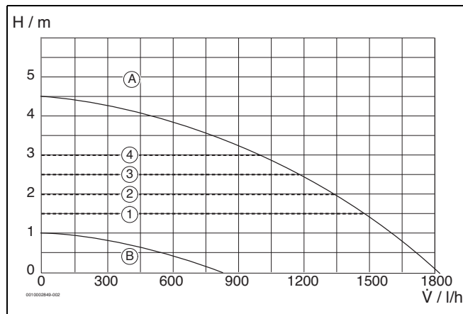
Bild 226 Pumpenkennfelder und Pumpenkennlinien
