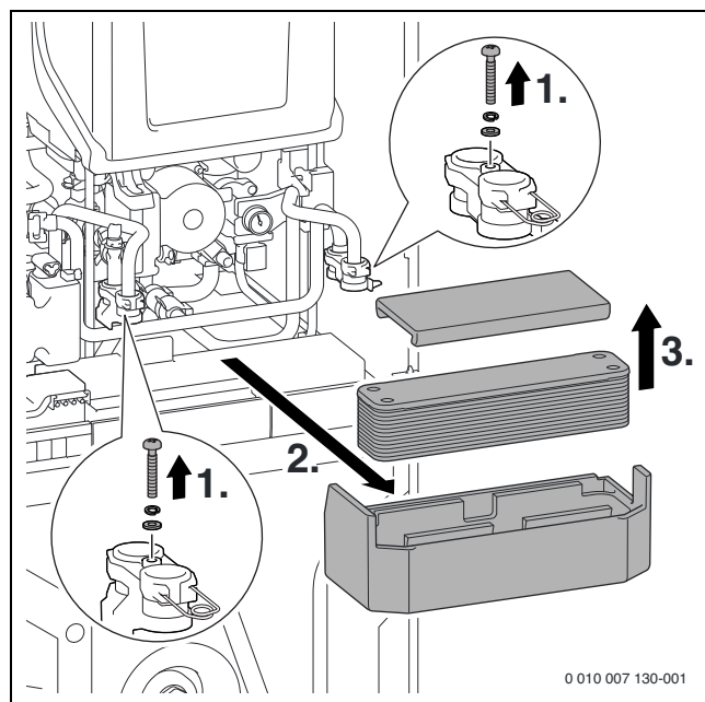
Bild 216 Plattenwärmetauscher ausbauen
