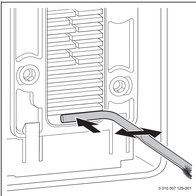
Bild 211 Kondensatwanne reinigen
