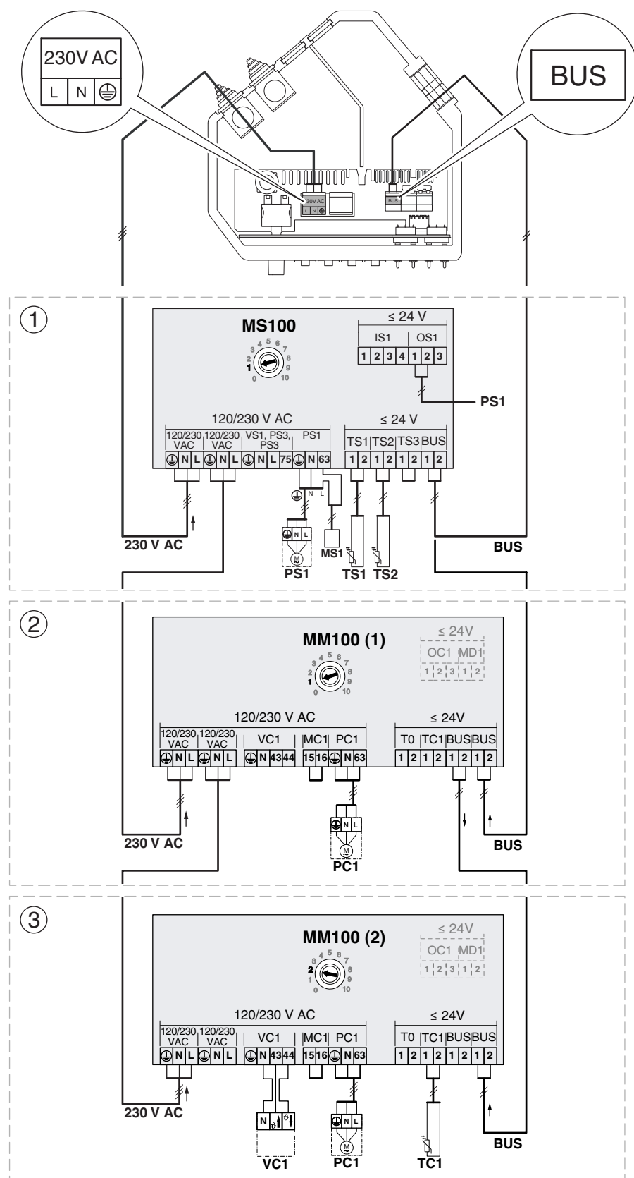
Bild 180 Anschluss der Module MS100 und MM100, wenn vorhanden
