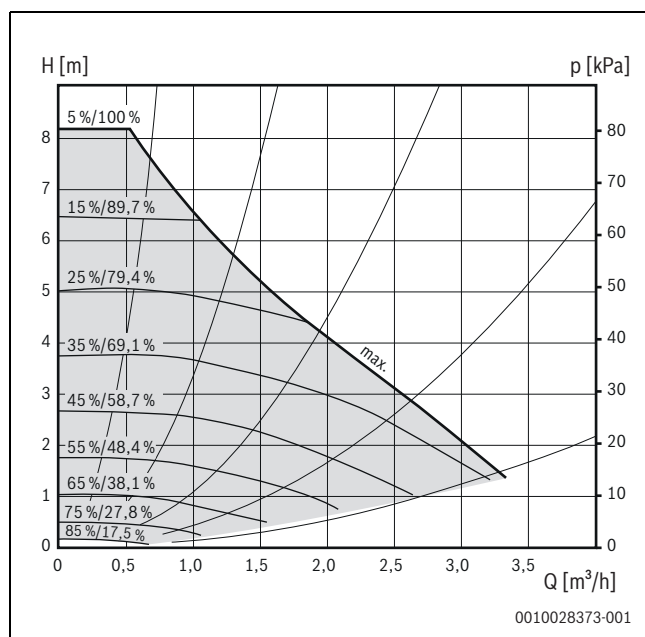
Bild 227 Pumpenkennfelder und Pumpenkennlinien der Solarpumpe Wilo Para ST 15/7-50/iPWM 2, Drehzahlbereich 20–100 %, Volumenstrombereich 0–16,5 l/min
