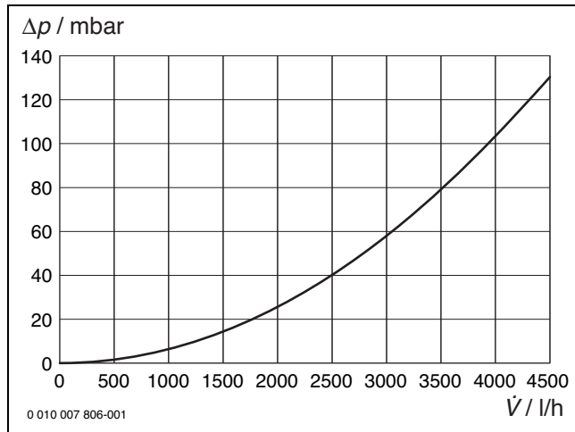
Bild 228 Druckverlust-Diagramm ungemischter Heizkreis (HK1)
