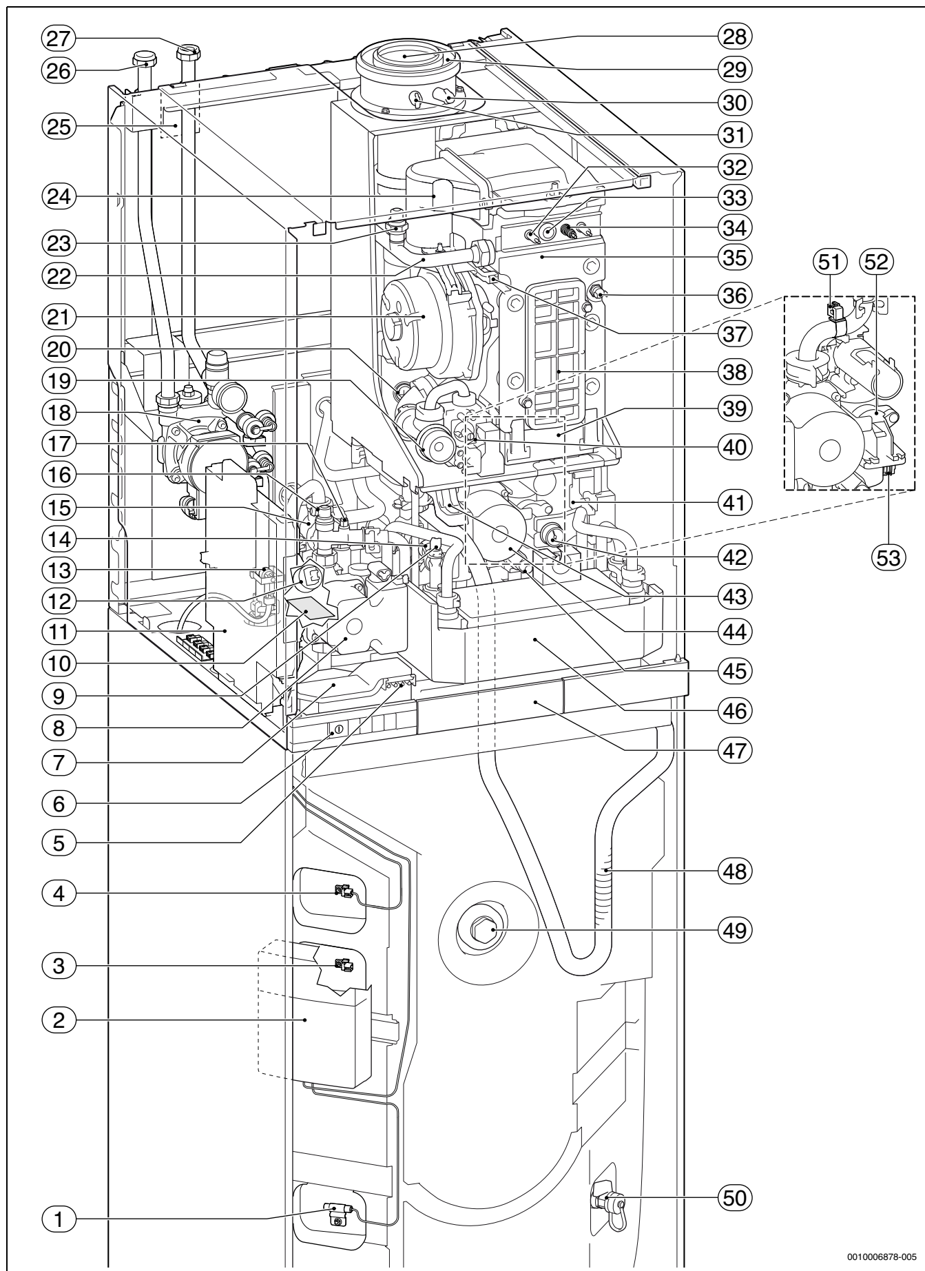
Bild 12 GB192... iT210...-Geräte
