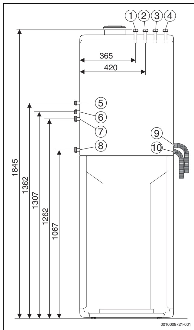
Bild 7 Anschlussmaße des Zubehörs Heizkreiserweiterung 1 (Maße in mm)
