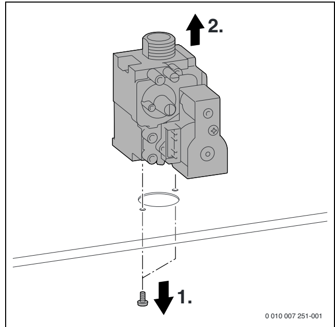
Bild 220 Gasarmatur ausbauen
