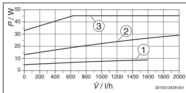
Bild 234 Leistungsaufnahme für die Pumpenstufen I bis III
