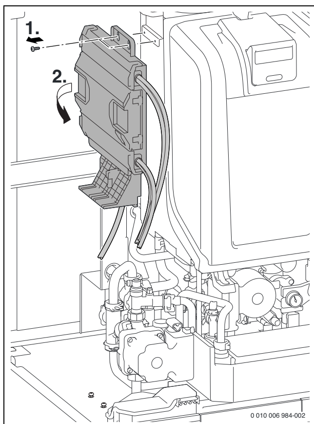
Bild 55 Steuergerät abnehmen
