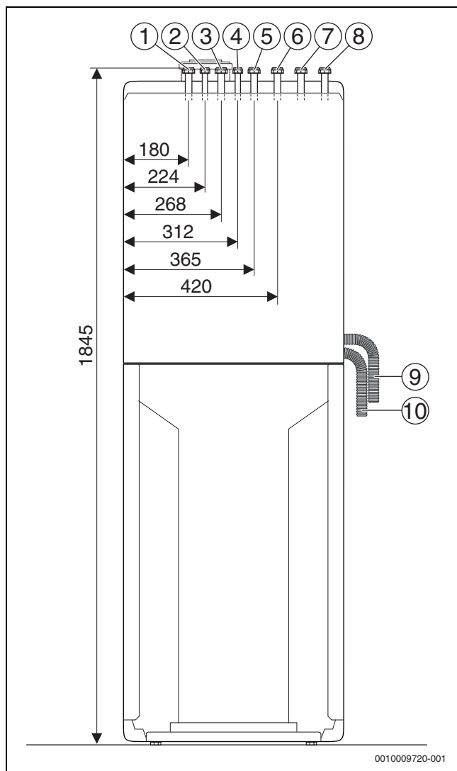
Bild 5 Anschlussmaße des Zubehörs AS-V1/Vertikales Anschluss-Set (Maße in mm)
