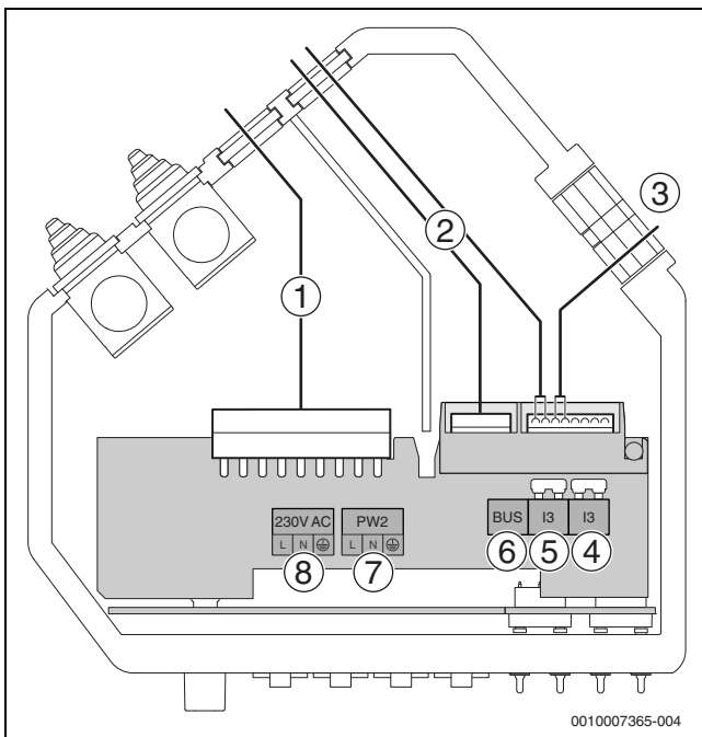
Bild 179 Anschlussbox
