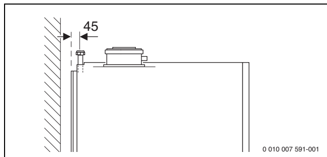
Bild 6 Anschlussmaße des Zubehörs AS-V1/Vertikales Anschluss-Set (Maße in mm)
