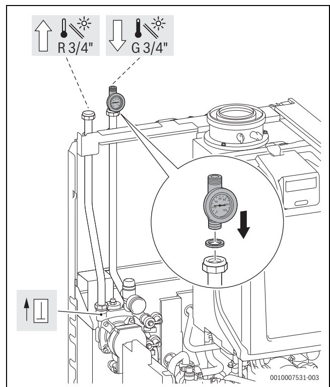
Bild 71 Wartungshahn mit Thermometer am Solar-Vorlaufrohr montieren
