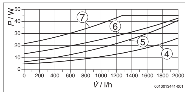
Bild 235 Leistungsaufnahme für Proportionaldruck und Konstantdruck
