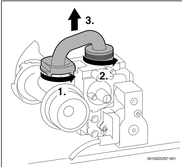
Bild 218 Gasrohr ausbauen
