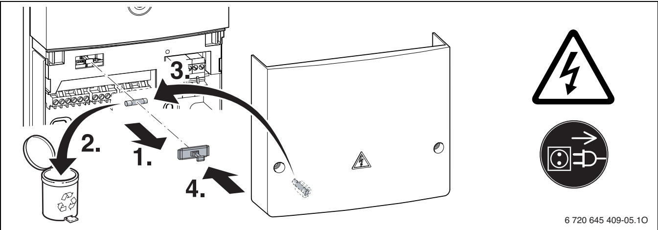
Bild 224 Sicherung vom Modul tauschen
