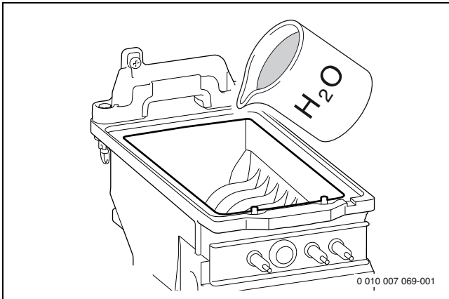
Bild 210 Spülen
