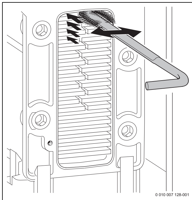
Bild 209 Wärmeblock mit Bürste reinigen
