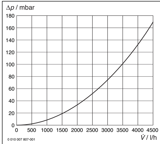
Bild 229 Druckverlust-Diagramm gemischter Heizkreis (HK2)
