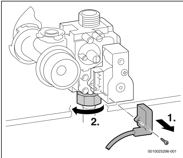
Bild 219 Stecker abziehen und Überwurfmutter lösen
