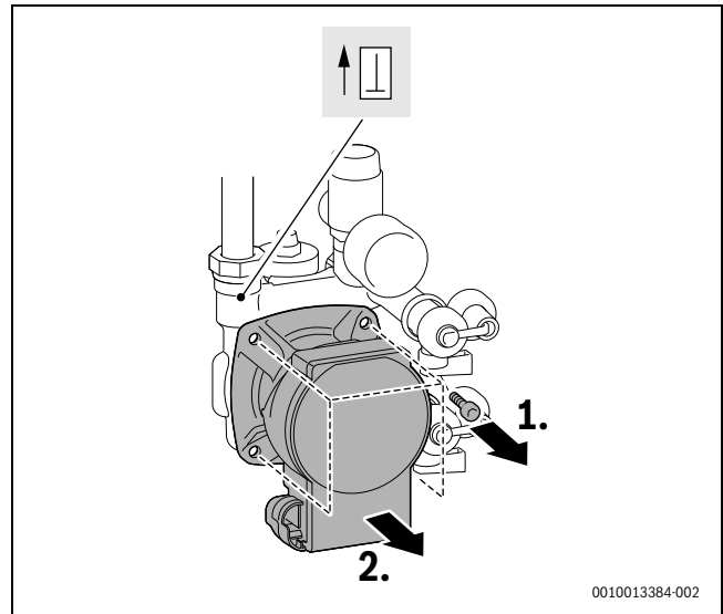
Bild 221 Solarpumpe ausbauen
