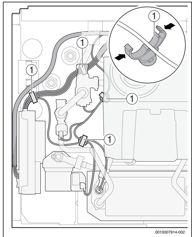
Bild 62 Kabel mit 4 Clips befestigen
