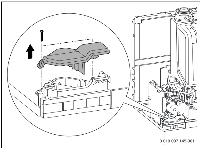
Bild 177 Abdeckung der Anschlussbox entfernen
