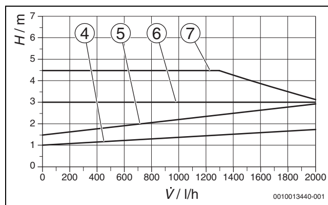
Bild 233 Pumpenkennlinien für Proportionaldruck und Konstantdruck
