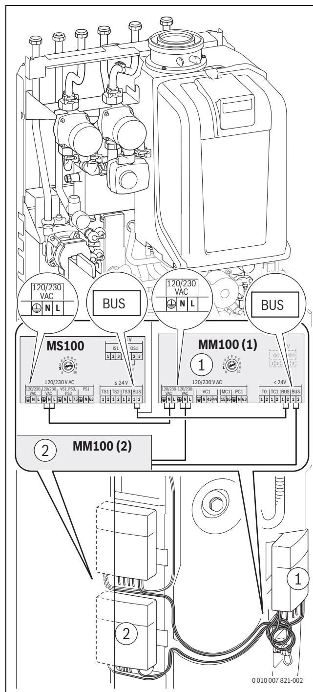
Bild 141 Anschluss am Modul MS100 und am Modul MM100 durchschleifen
