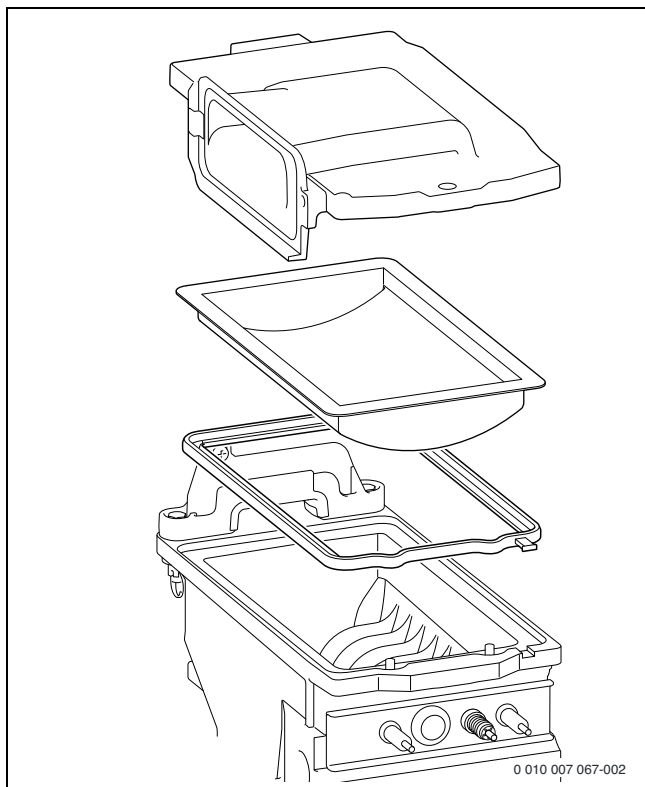
Bild 207 Brenner
