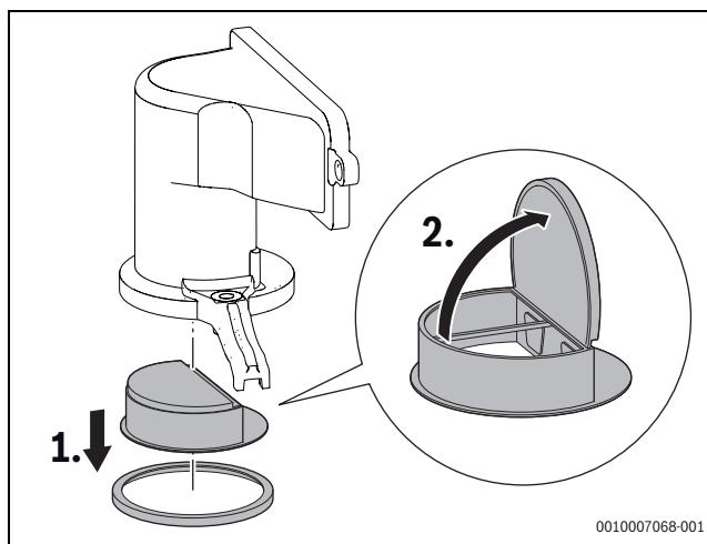
Bild 215 Rückschlagklappe in der Mischeinrichtung
