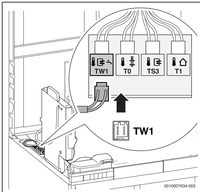
Bild 59 Speichertemperaturfühler anschließen
