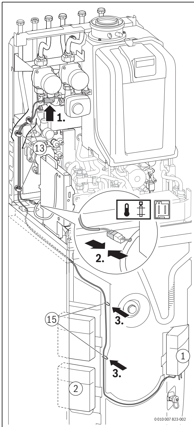
Bild 136 Anschluss Heizungspumpe ungemischter Heizkreis und Hyd- raulische Weiche
