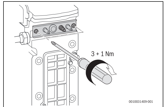
Bild 204 Elektroden-Set wieder einbauen
