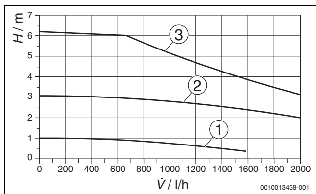
Bild 232 Pumpenkennlinien für die Pumpenstufen I bis III
