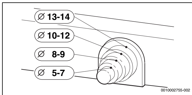
Bild 139 Zugentlastung Kabel Mischermotor anpassen
