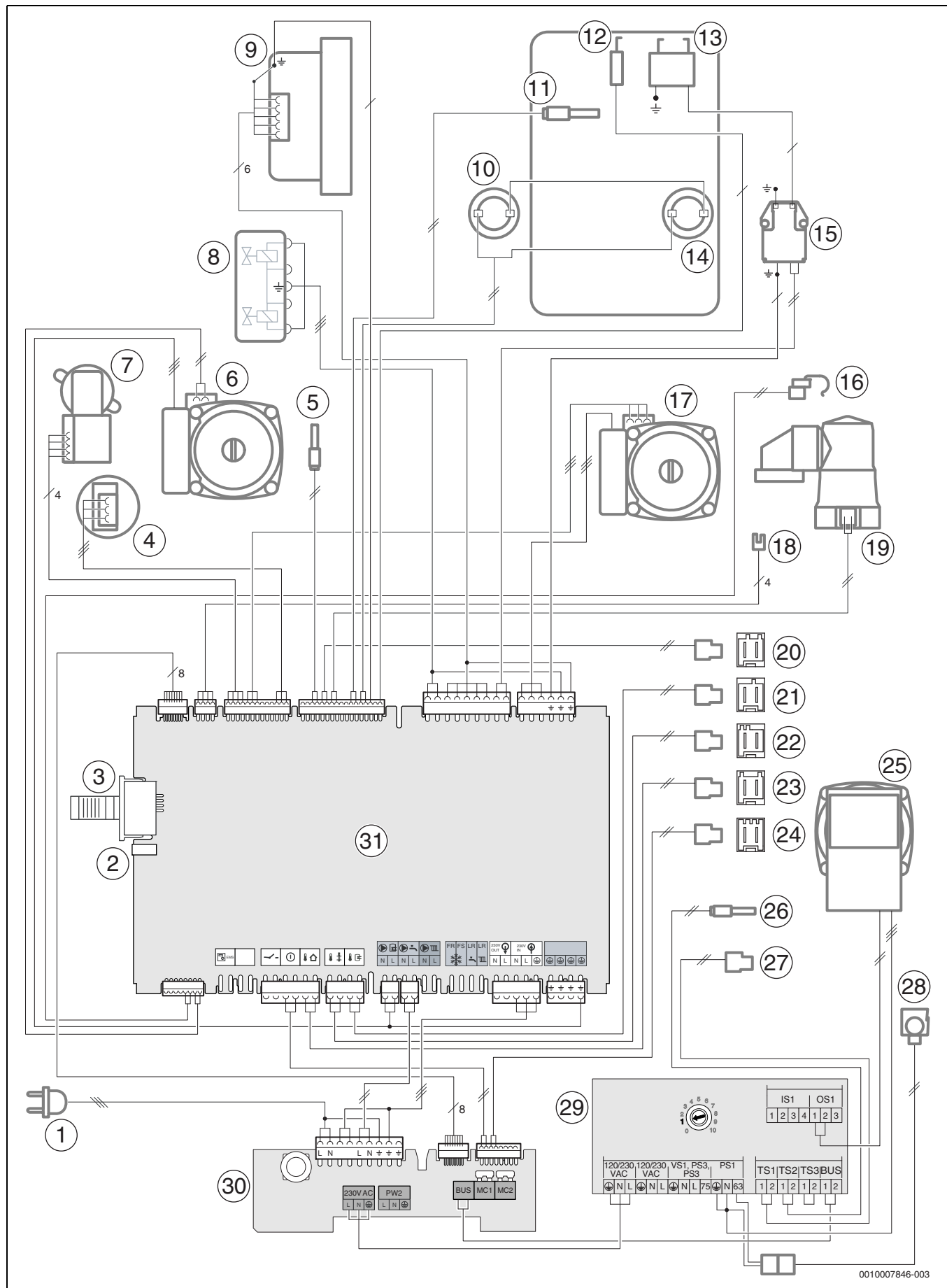
Bild 225 Elektrische Verdrahtung
