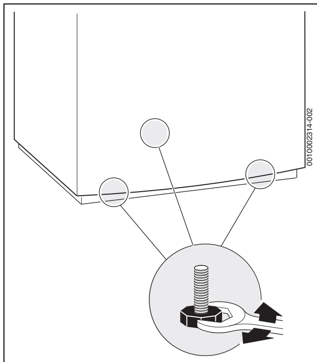
Bild 46 Speicher ausrichten
