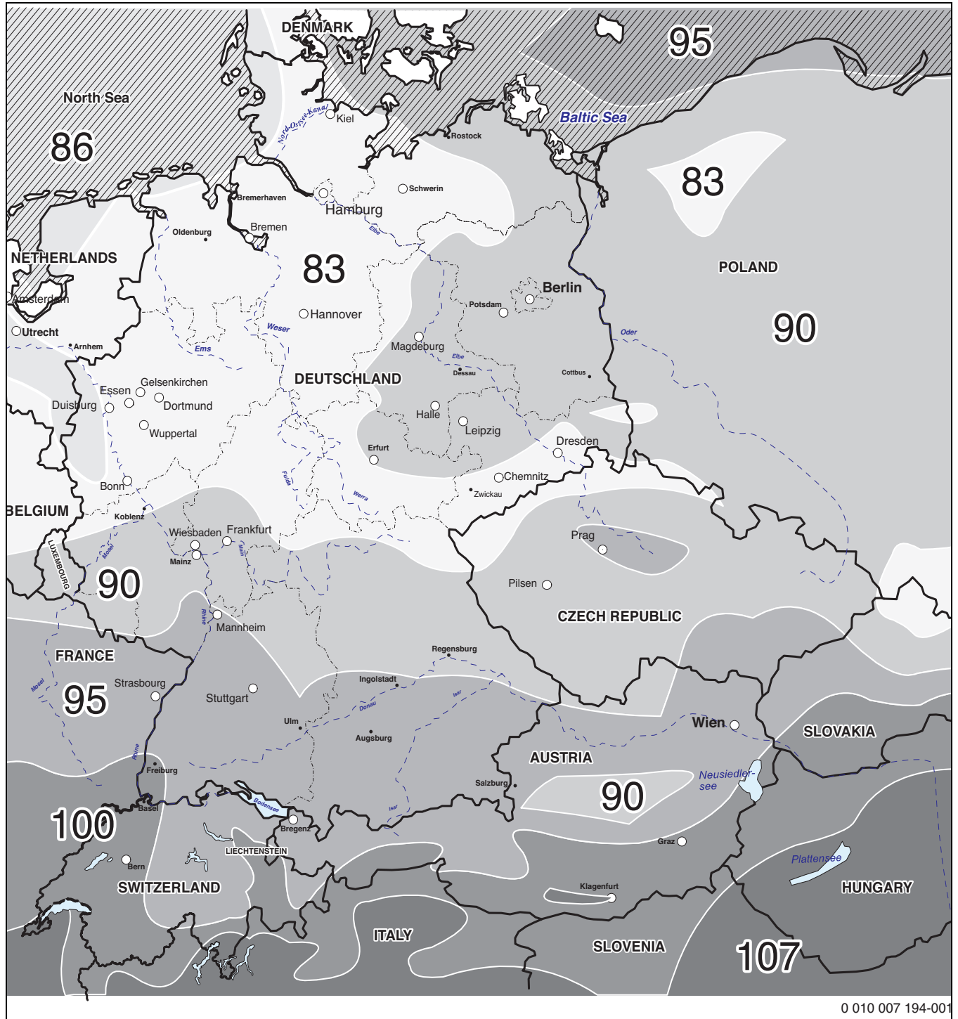
Bild 236 Übersicht der Klimazonen
