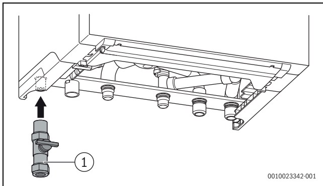
Bild 13 Gasanschluss herstellen
