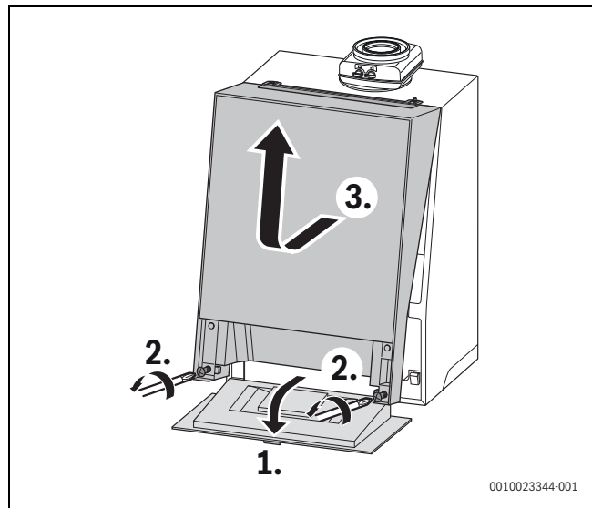
Bild 14 Verkleidung Gerät demontieren
