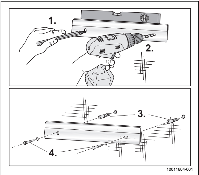
Bild 11 Aufhängeschiene montieren
