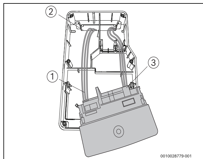
Bild 51 Funktionsmodul anschließen
