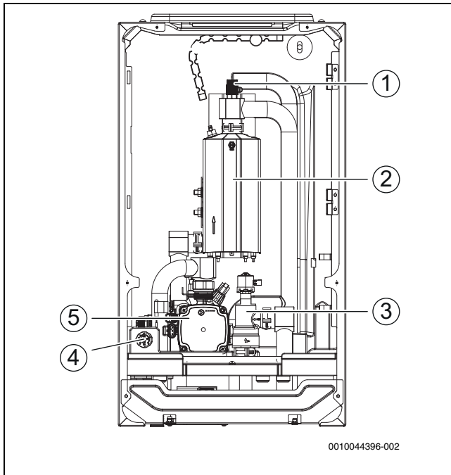
Bild 5 Komponenten
