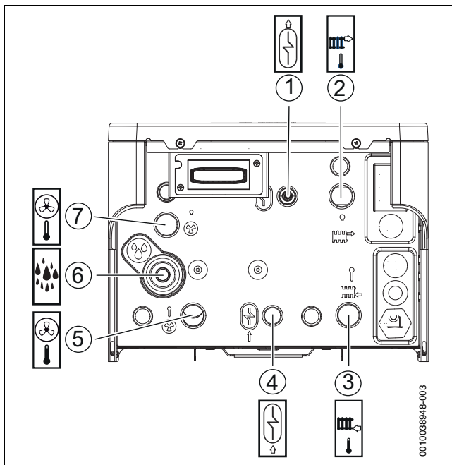
Bild 6 Rohranschlüsse
