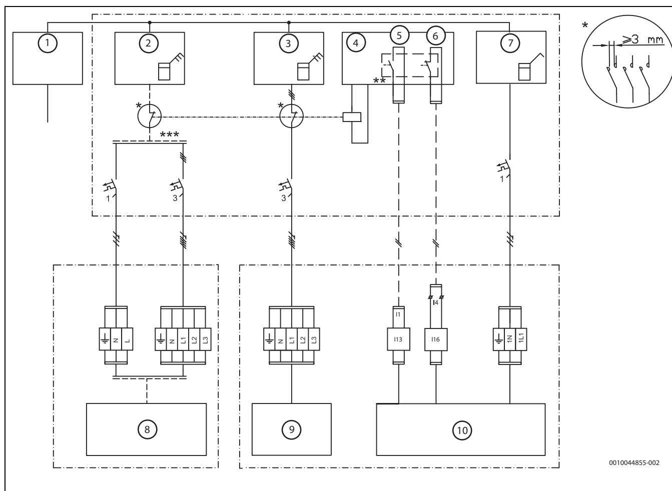
Bild 42 Alternative Lösung
