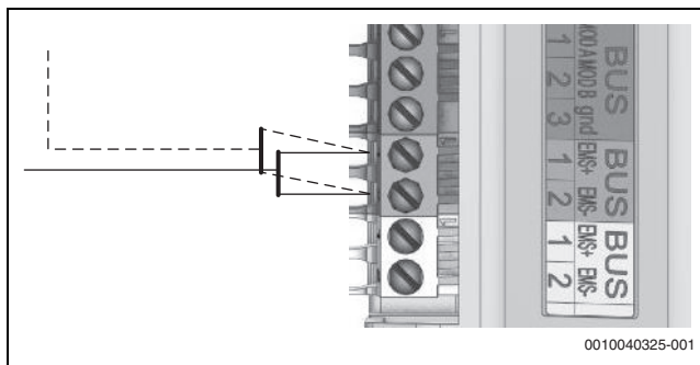
Bild 26 EMS-Anschluss
